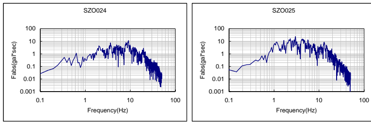
図 A2.6(3) フーリエスペクトル一覧 (2001年2月23日 静岡県西部地震)
