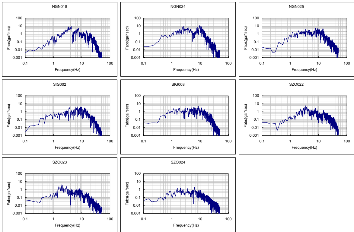
図 A2.7(3) フーリエスペクトル一覧 (2001年1月6日 岐阜県美濃東部地震)
