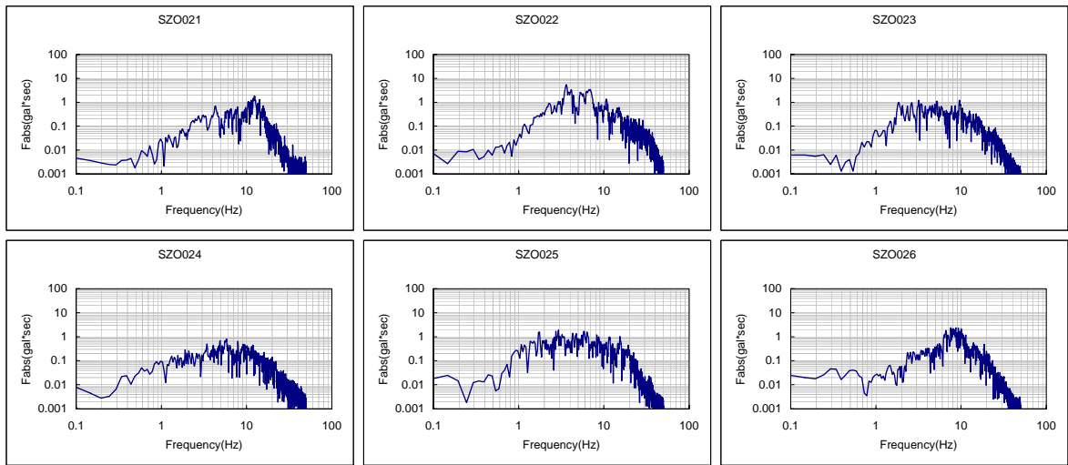
図 A2.2(3) フーリエスペクトル一覧 (2002年4月11日 愛知県西部地震)
