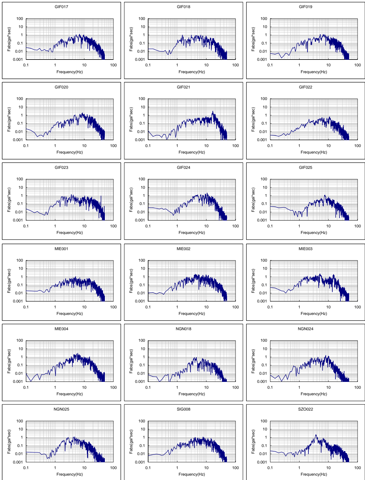
図 A2.4(2) フーリエスペクトル一覧 (2001年9月22日 愛知県西部地震)
