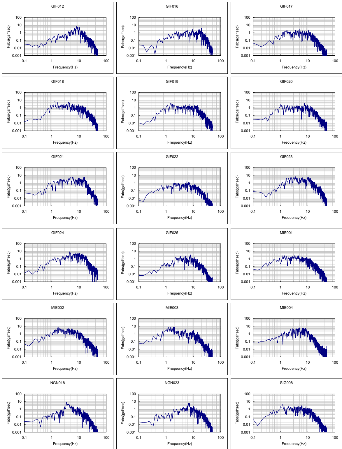
図 A2.6(2) フーリエスペクトル一覧 (2001年2月23日 静岡県西部地震)
