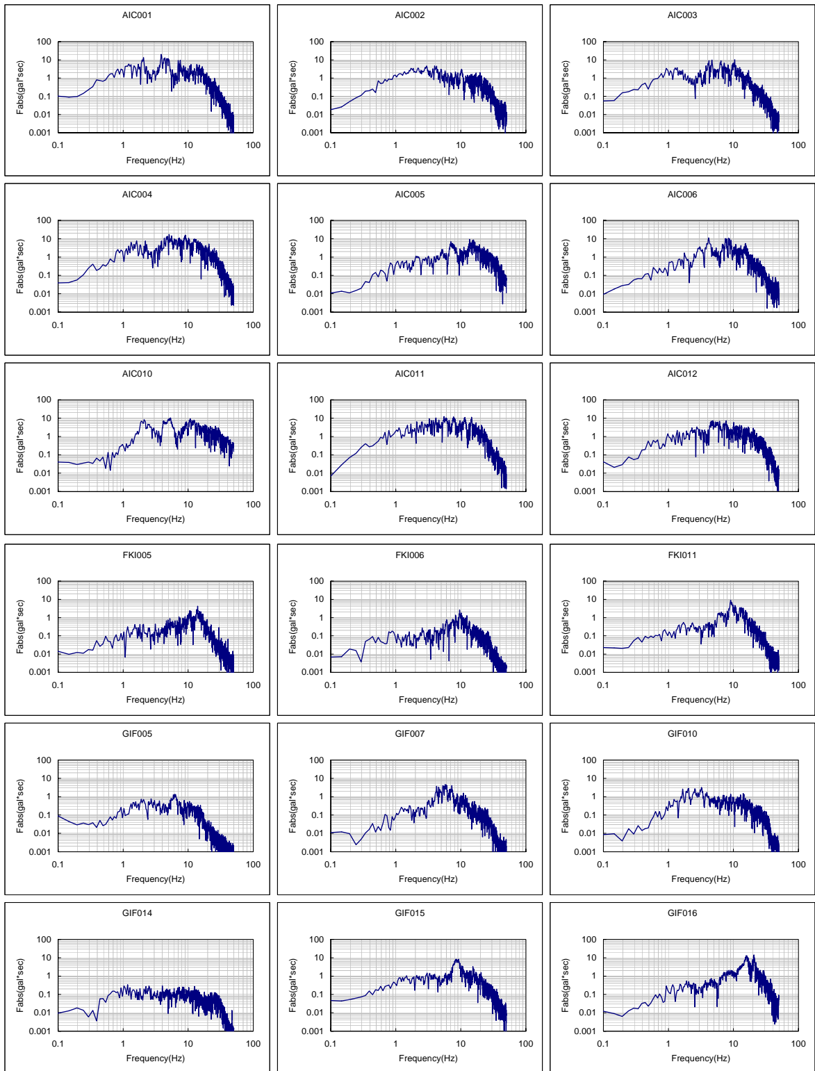
図 A2.11(1) フーリエスペクトル一覧 (1999年11月29日 愛知県西部地震)
