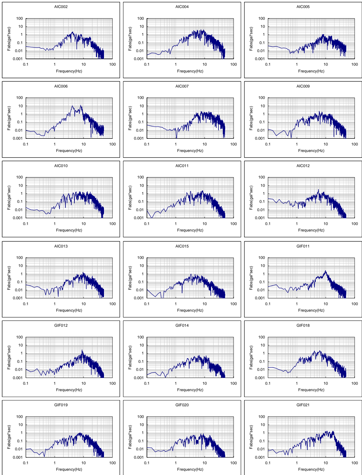
図 A2.9(1) フーリエスペクトル一覧 (2000年7月20日 愛知県西部地震)
