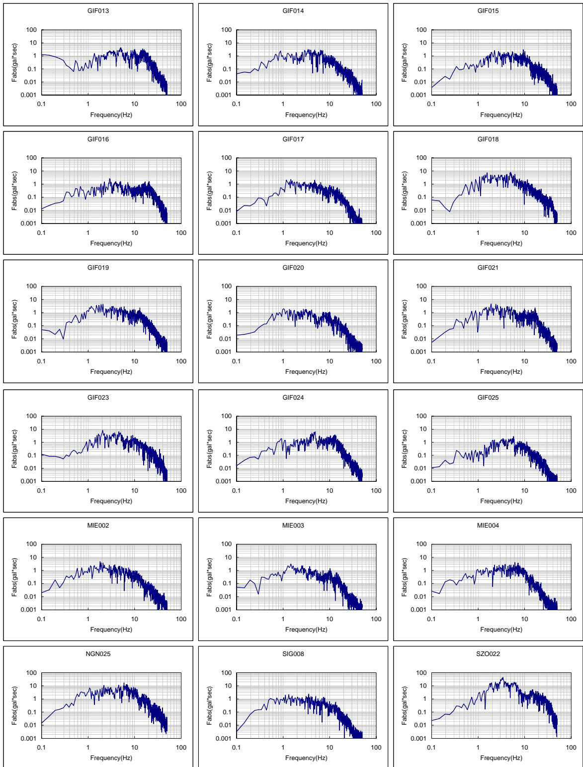
図 A2.5(2) フーリエスペクトル一覧 (2001年4月3日 静岡県中部地震)
