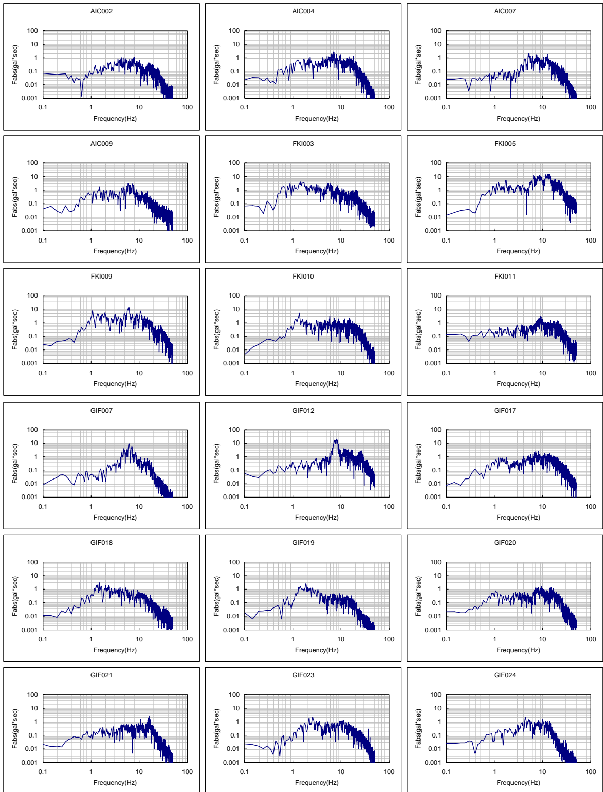
図 A2.10(1) フーリエスペクトル一覧 (2000年6月5日 福井県嶺南地震)
