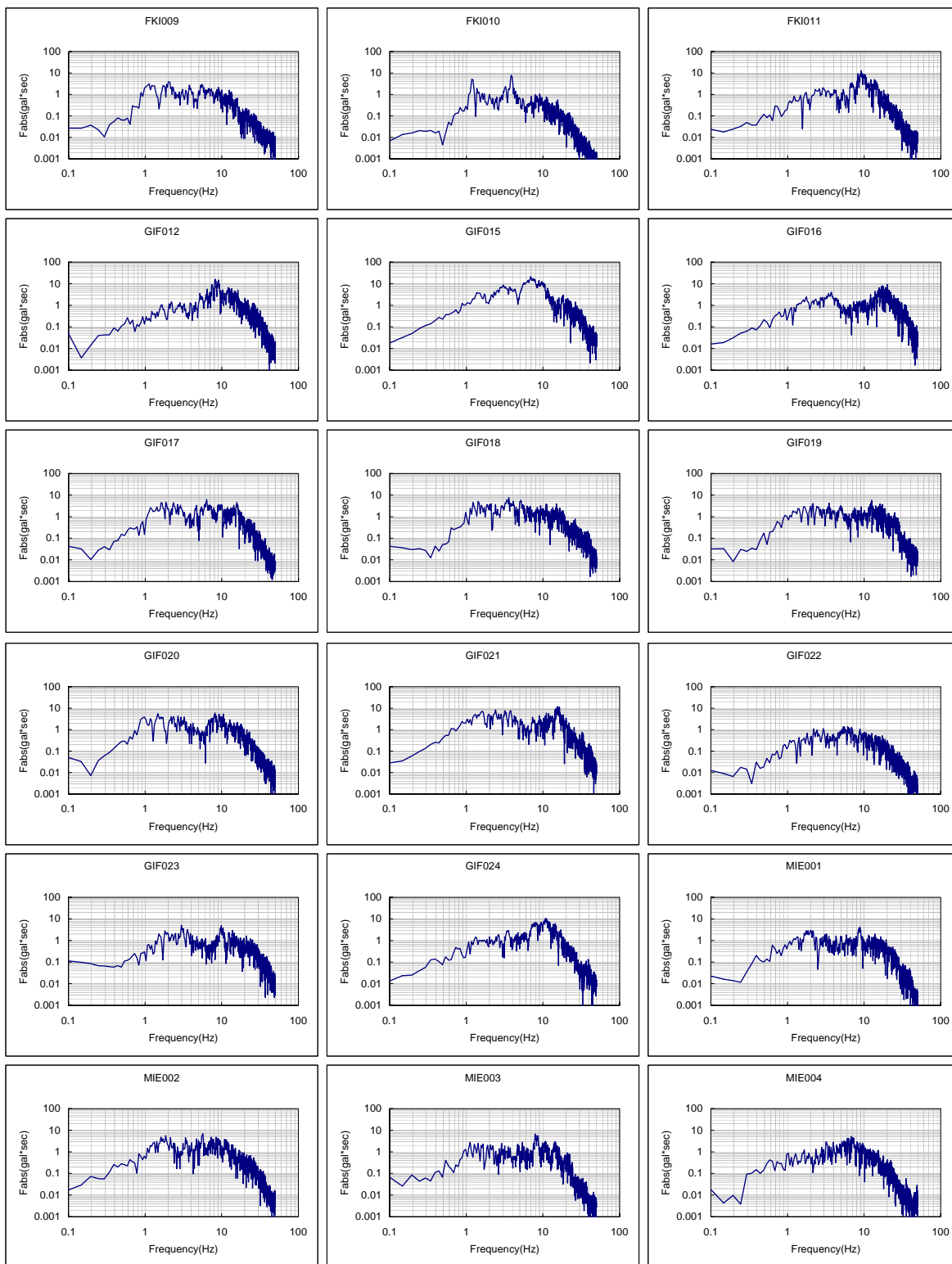
図 A2.7(2) フーリエスペクトル一覧 (2001年1月6日 岐阜県美濃東部地震)
