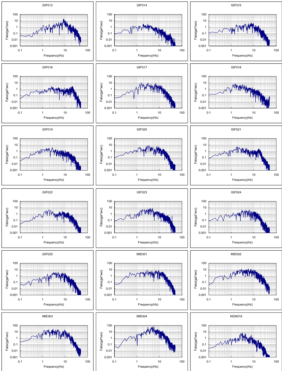
図 A2.8(2) フーリエスペクトル一覧 (2000年10月31日 三重県南部地震)
