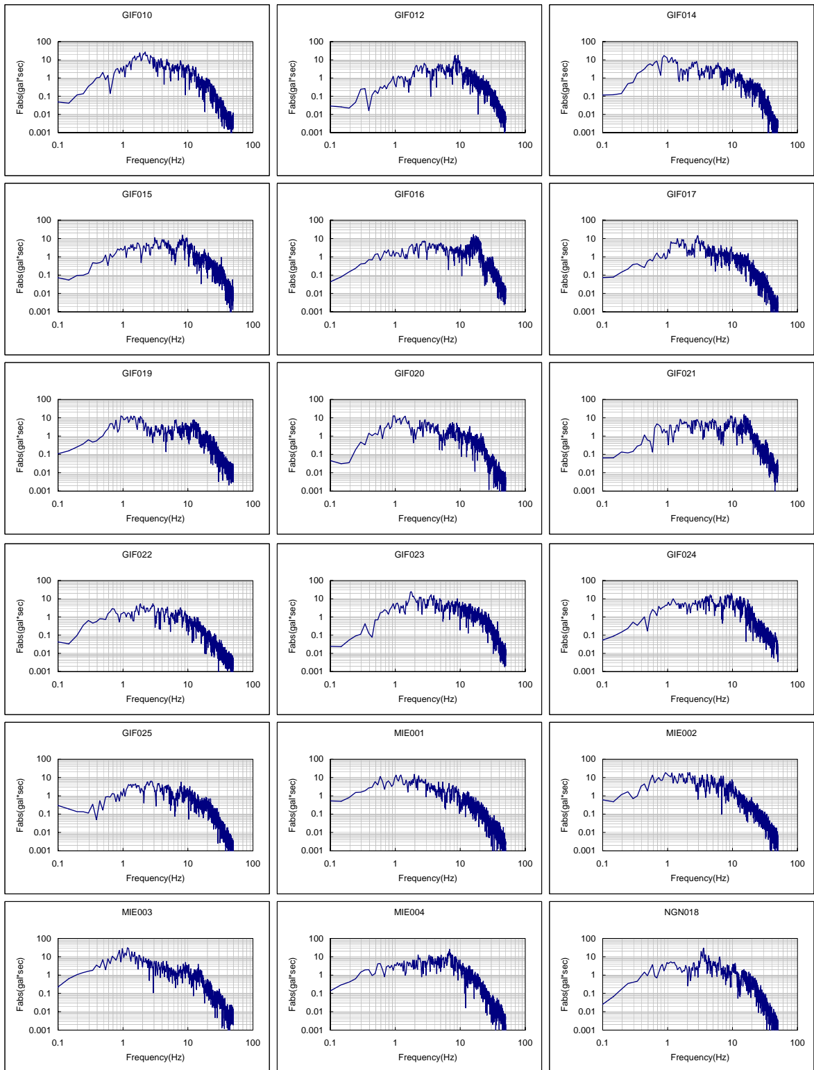
図 A2.16(2) フーリエスペクトル一覧 (1997年3月16日 愛知県東部地震)
