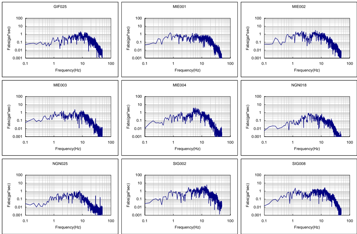
図 A2.10(2) フーリエスペクトル一覧 (2000年6月5日 福井県嶺南地震)
