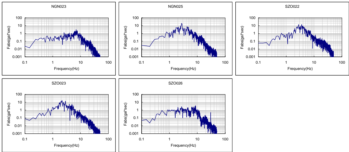
図 A2.8(3) フーリエスペクトル一覧 (2000年10月31日 三重県南部地震)
