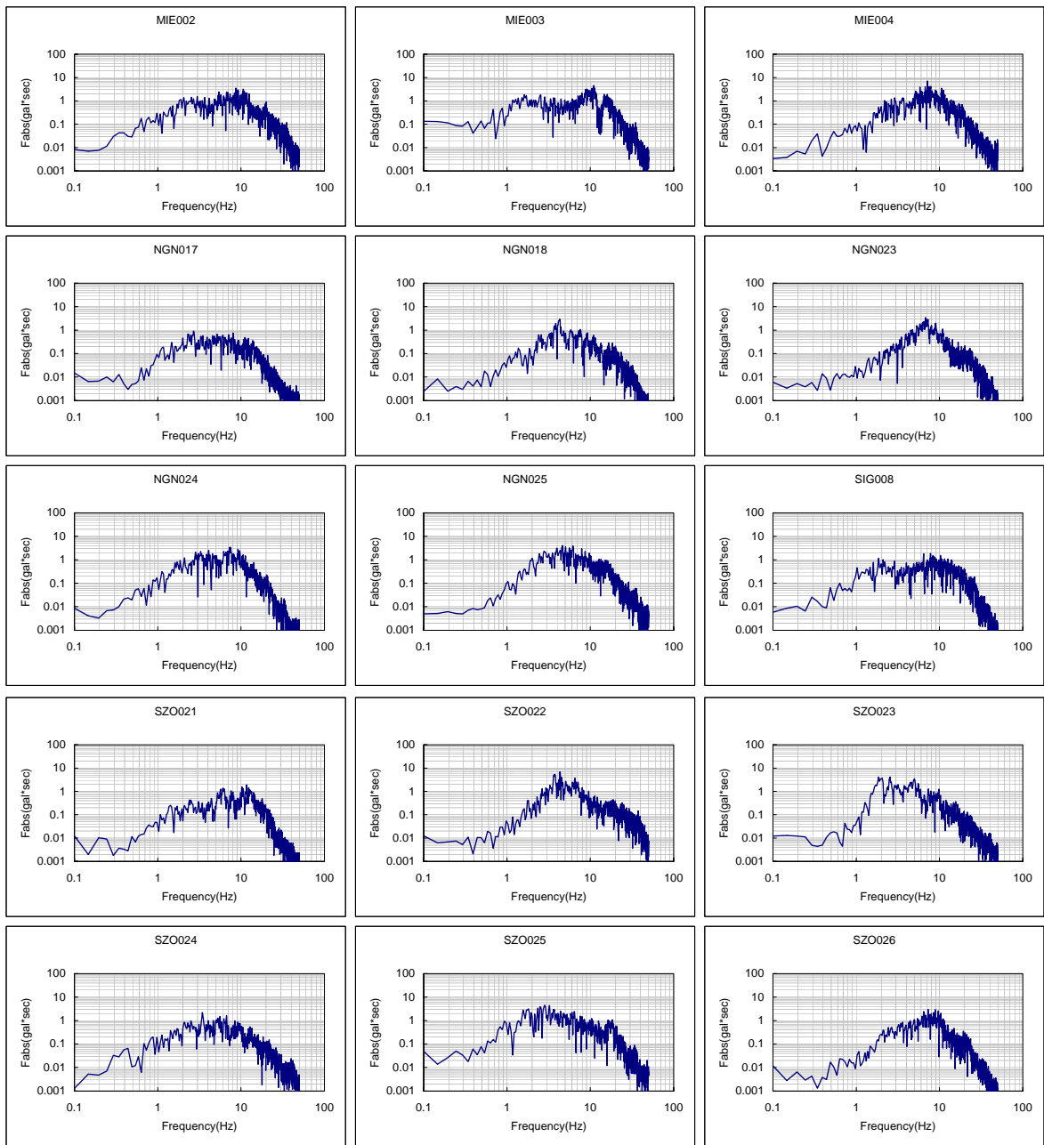
図 A2.3(3) フーリエスペクトル一覧 (2001年9月27日 愛知県西部地震)
