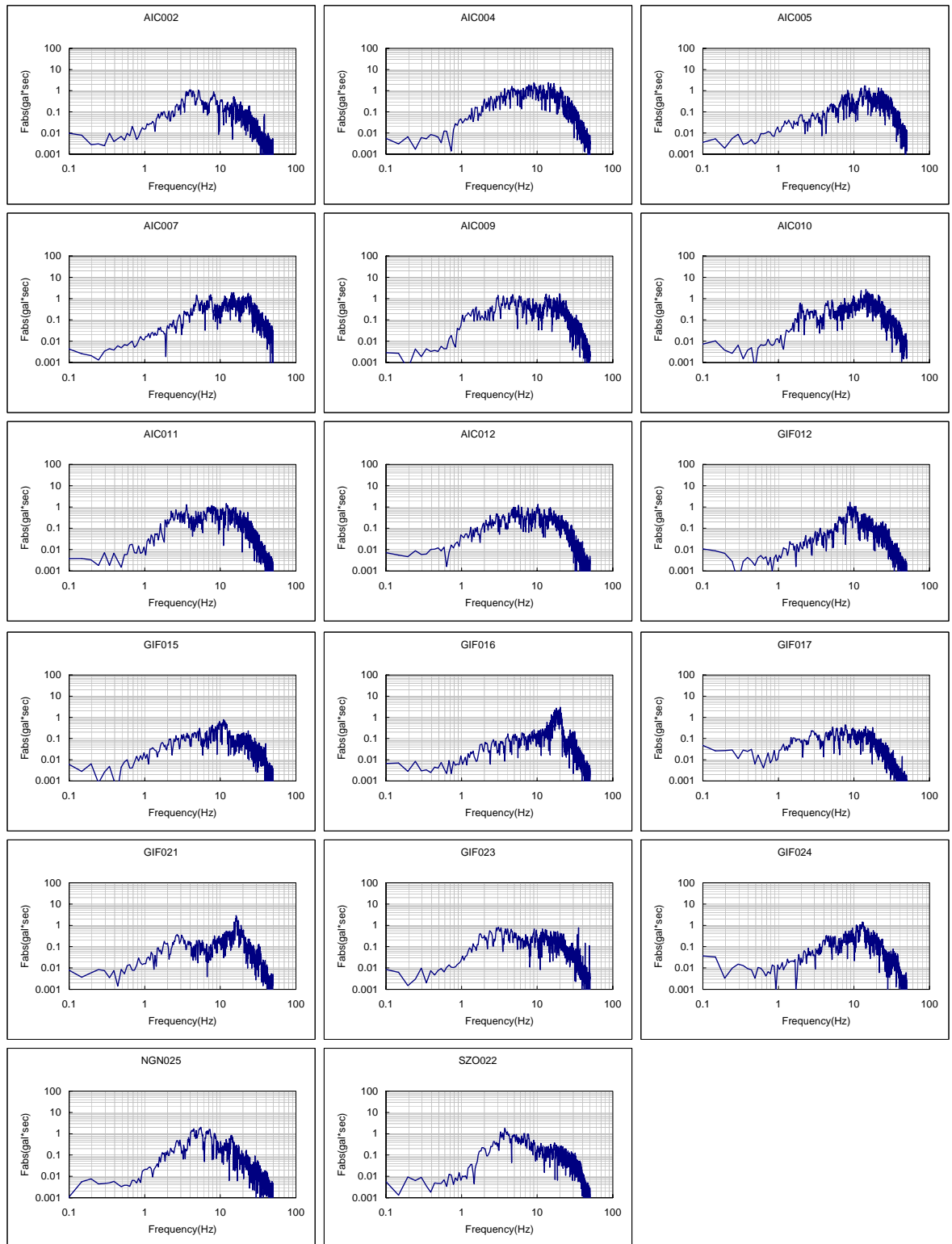
図 A2.13(1) フーリエスペクトル一覧 (1998 年 4 月 25 日 愛知県東部地震)
