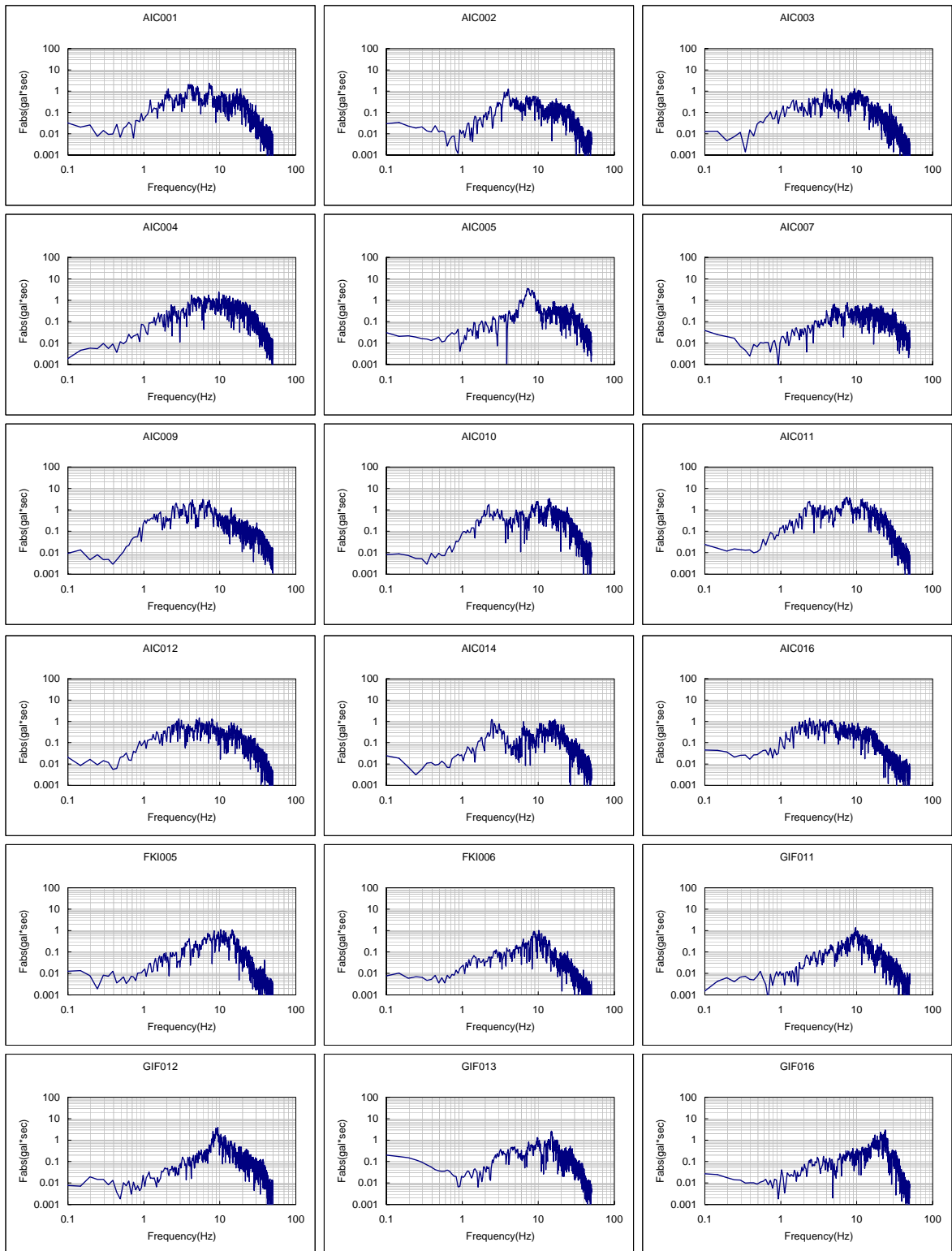
図 A2.4(1) フーリエスペクトル一覧 (2001年9月22日 愛知県西部地震)
