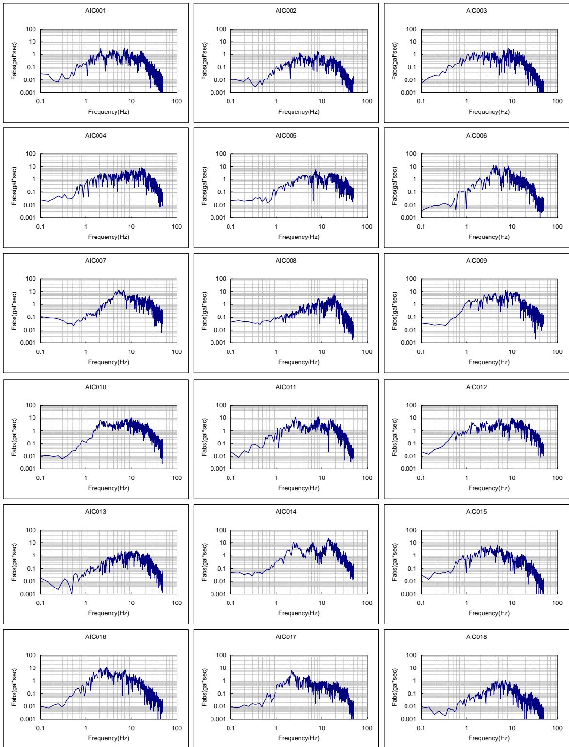
図 A2.3(1) フーリエスペクトル一覧 (2001年9月27日 愛知県西部地震)
