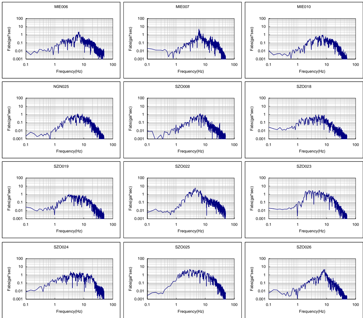
図 A2.1(2) フーリエスペクトル一覧 (2002年8月11日 静岡県西部地震)
