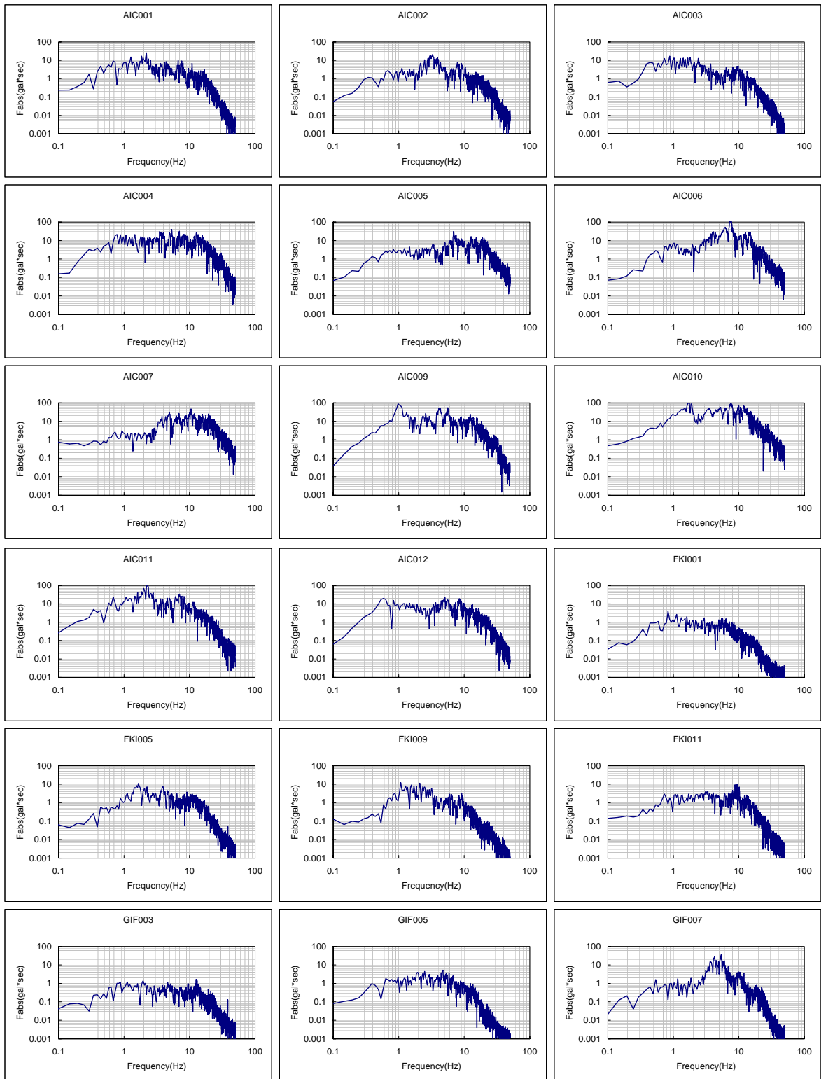
図 A2.16(1) フーリエスペクトル一覧 (1997年3月16日 愛知県東部地震)
