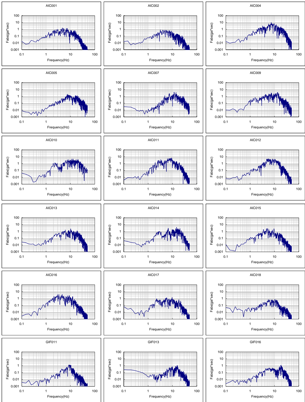
図 A2.2(1) フーリエスペクトル一覧 (2002年4月11日 愛知県西部地震)
