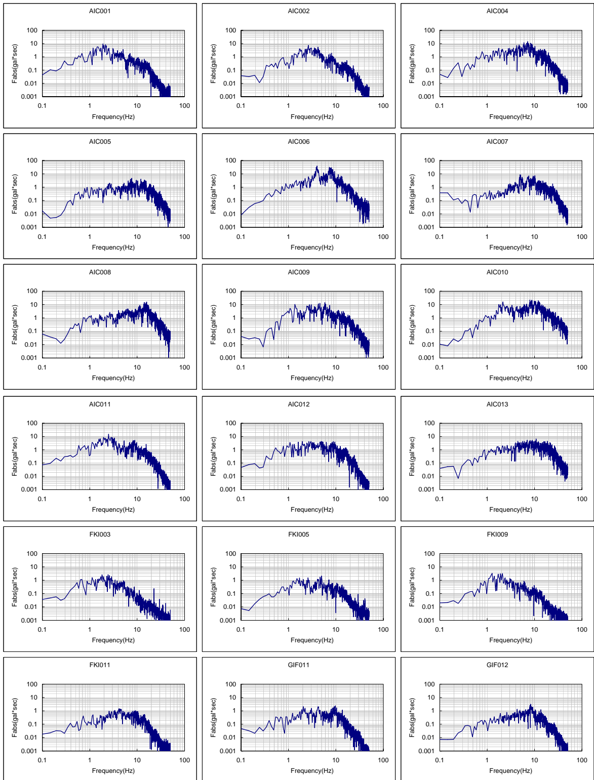
図 A2.5(1) フーリエスペクトル一覧 (2001年4月3日 静岡県中部地震)
