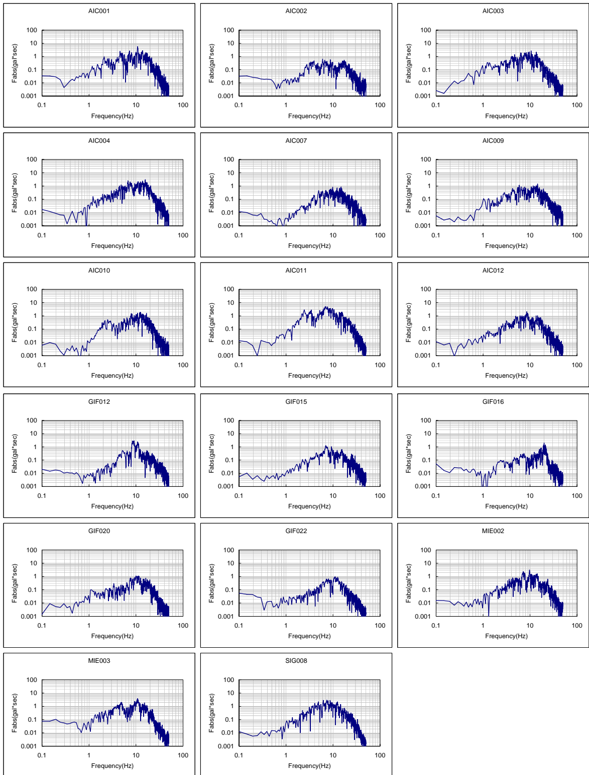
図 A2.12(1) フーリエスペクトル一覧 (1998 年 12 月 2 日 三重県北部地震)
