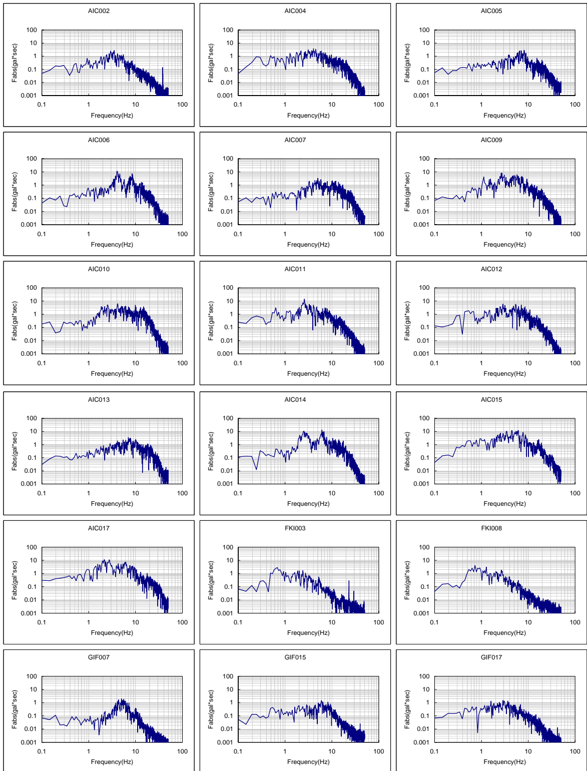
図 A2.15(1) フーリエスペクトル一覧 (1997年5月24日 遠州灘地震)
