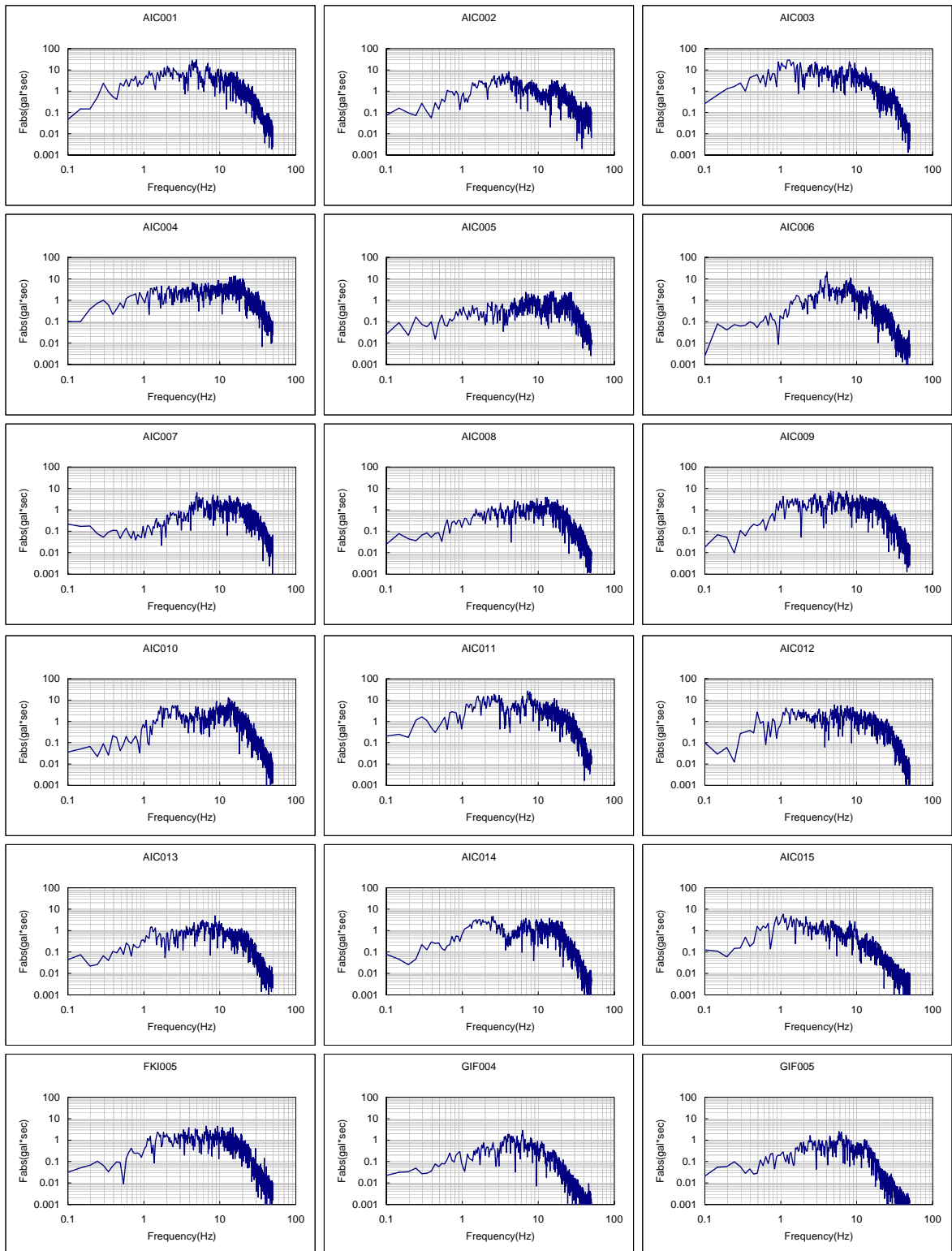
図 A2.14(1) フーリエスペクトル一覧 (1998年4月22日 岐阜県美濃中西部地震)
