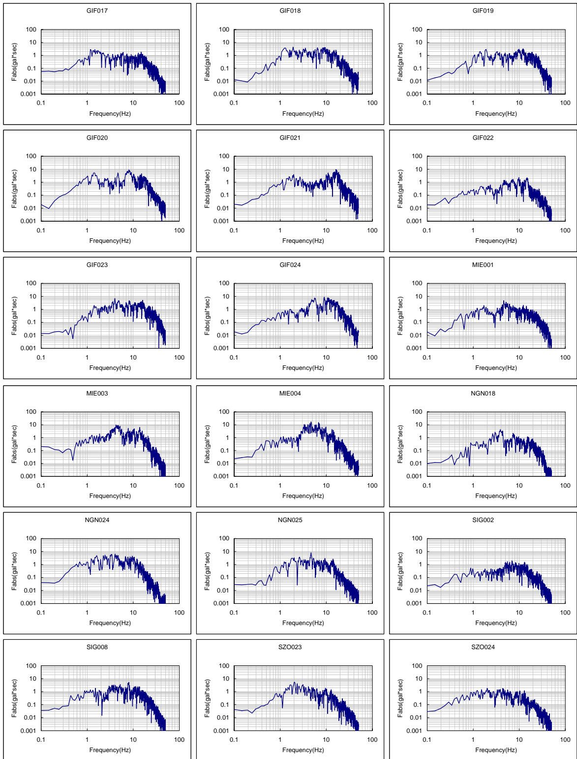
図 A2.11(2) フーリエスペクトル一覧 (1999年11月29日 愛知県西部地震)
