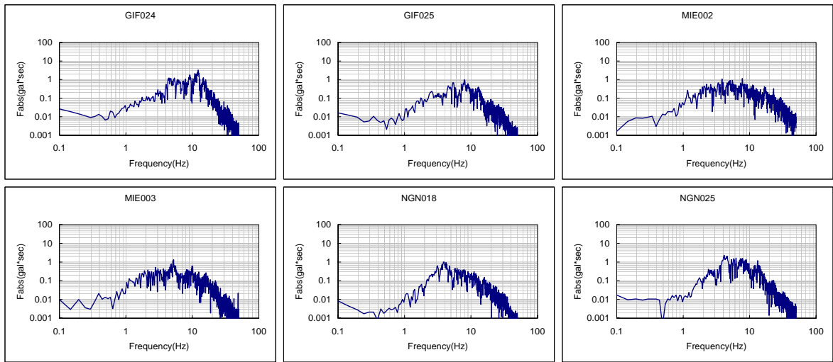
図 A2.9(2) フーリエスペクトル一覧 (2000年7月20日 愛知県西部地震)
