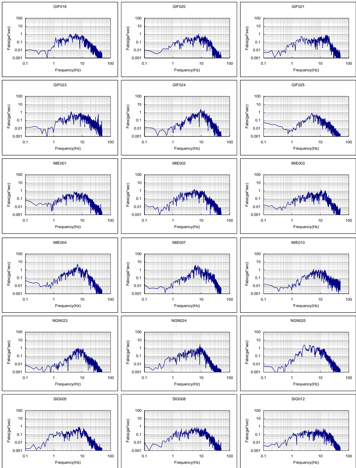
図 A2.2(2) フーリエスペクトル一覧 (2002年4月11日 愛知県西部地震)
