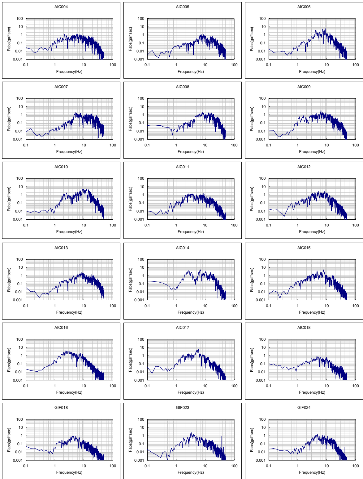
図 A2.1(1) フーリエスペクトル一覧 (2002年8月11日 静岡県西部地震)
