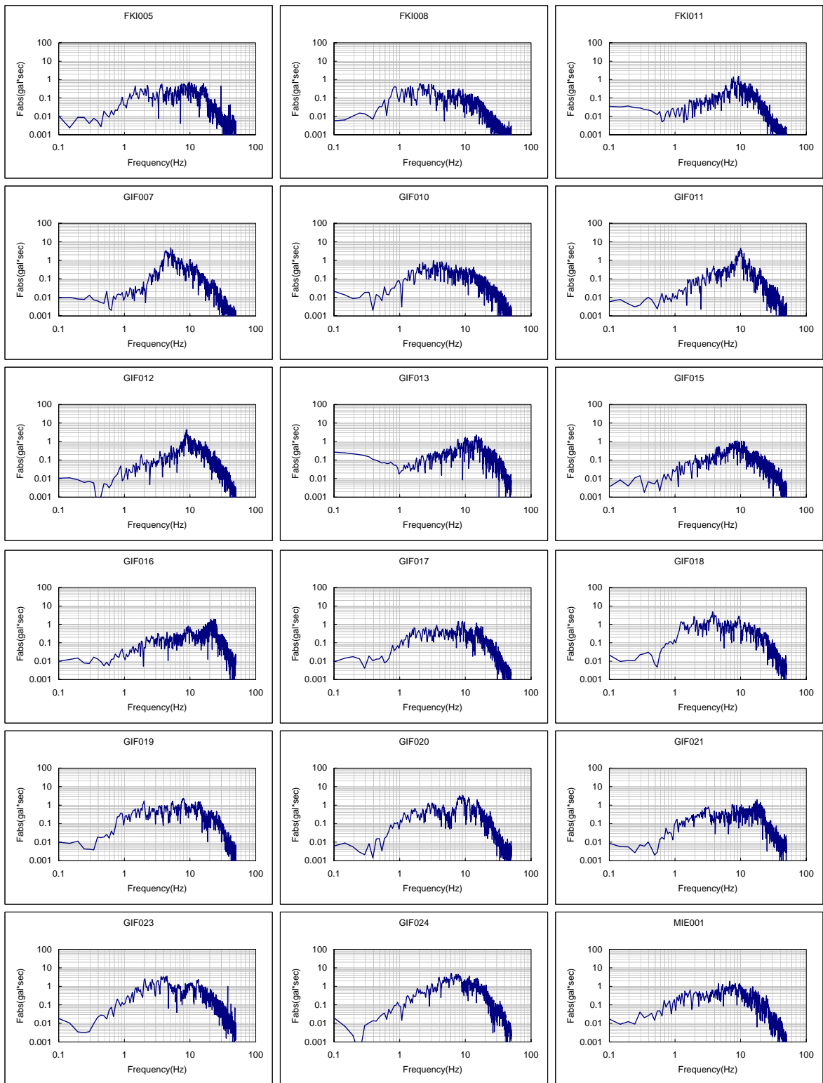
図 A2.3(2) フーリエスペクトル一覧 (2001年9月27日 愛知県西部地震)
