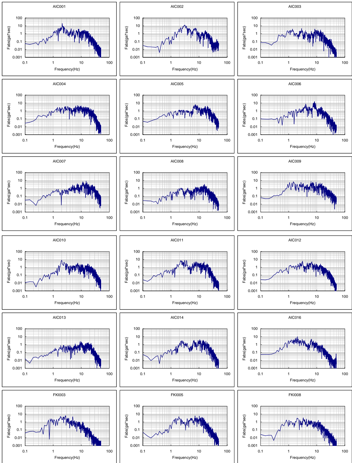
図 A2.7(1) フーリエスペクトル一覧 (2001年1月6日 岐阜県美濃東部地震)
