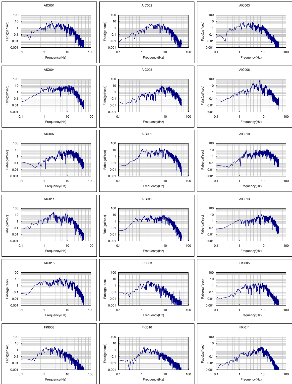
図 A2.6(1) フーリエスペクトル一覧 (2001年2月23日 静岡県西部地震)
