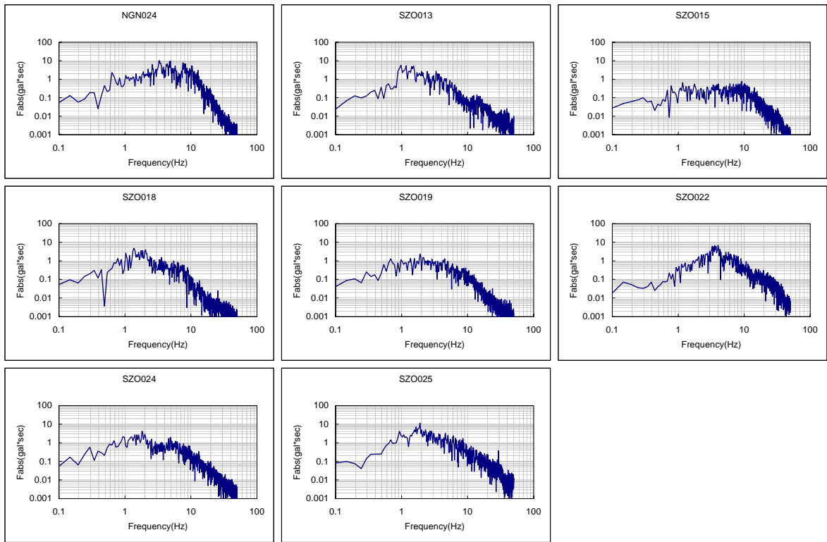
図 A2.14(3) フーリエスペクトル一覧 (1998年4月22日 岐阜県美濃中西部地震)
