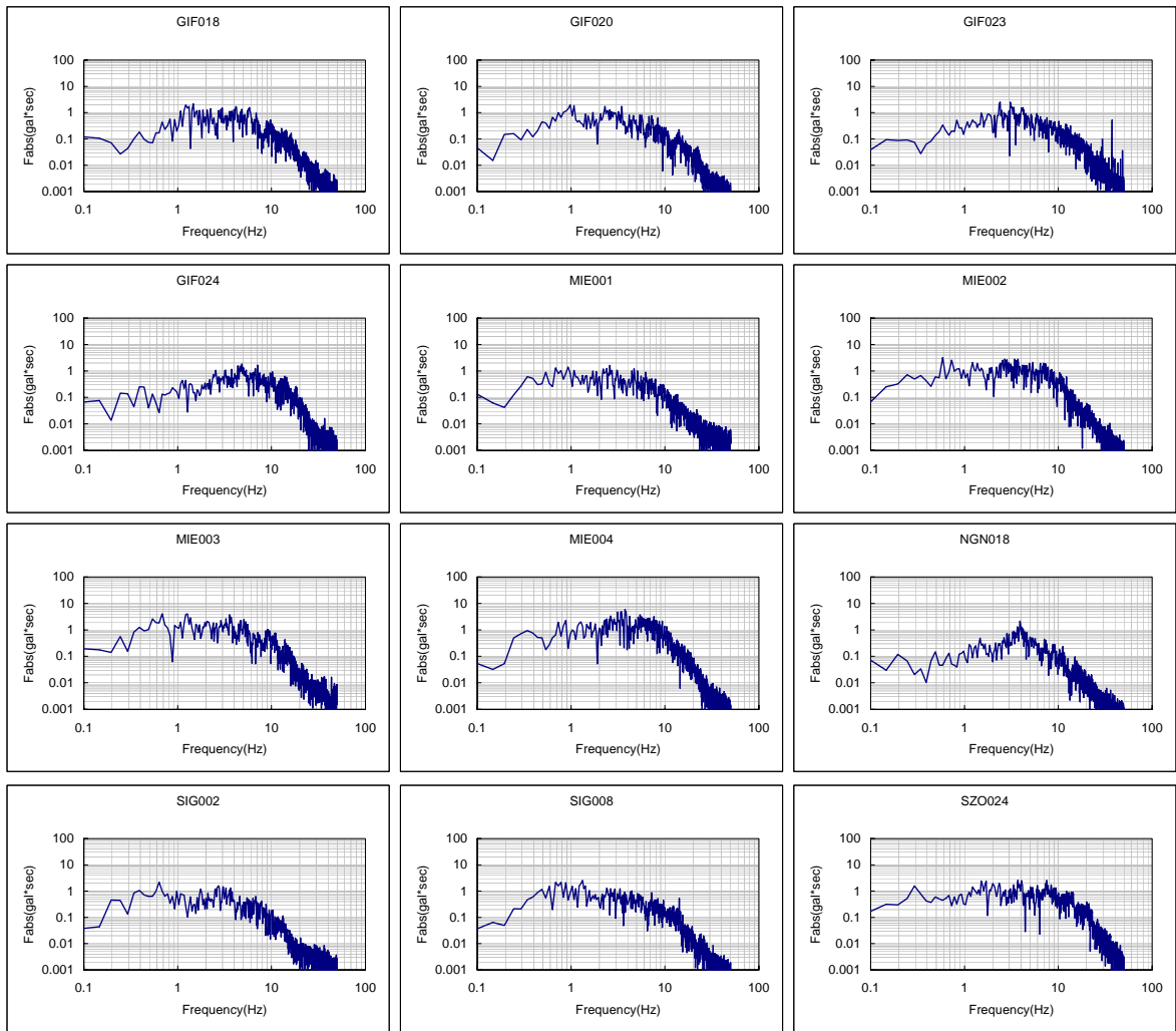
図 A2.15(2) フーリエスペクトル一覧 (1997年5月24日 遠州灘地震)
