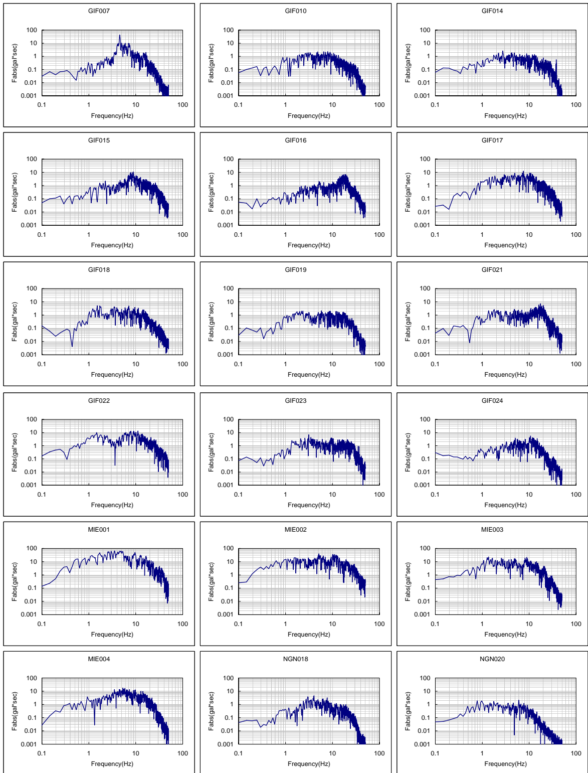
図 A2.14(2) フーリエスペクトル一覧 (1998年4月22日 岐阜県美濃中西部地震)
