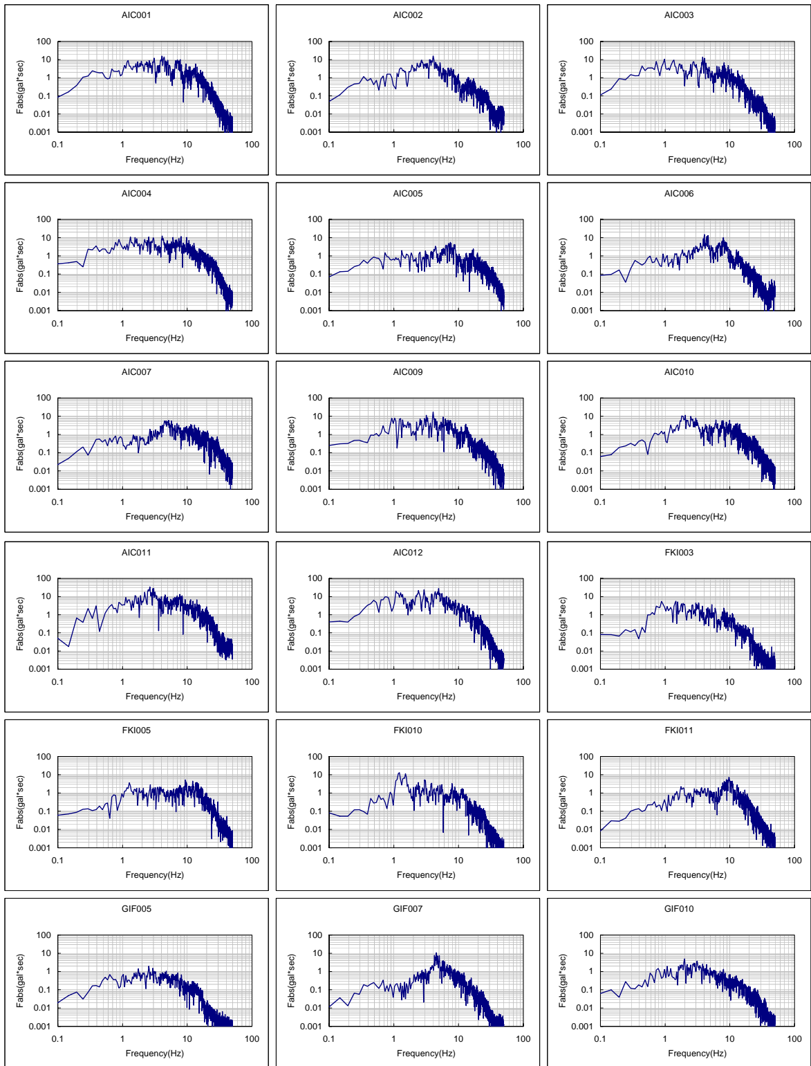
図 A2.8(1) フーリエスペクトル一覧 (2000年10月31日 三重県南部地震)
