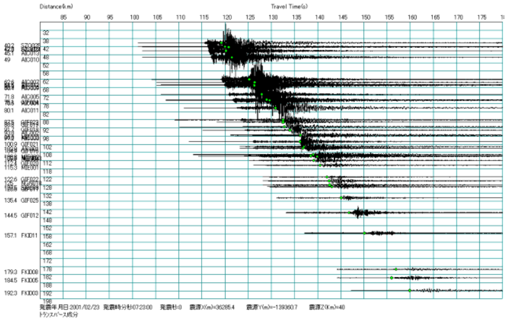
図 A1.15 トランスバースに変換した波形の一例 (1997年5月24日 遠州灘地震)
