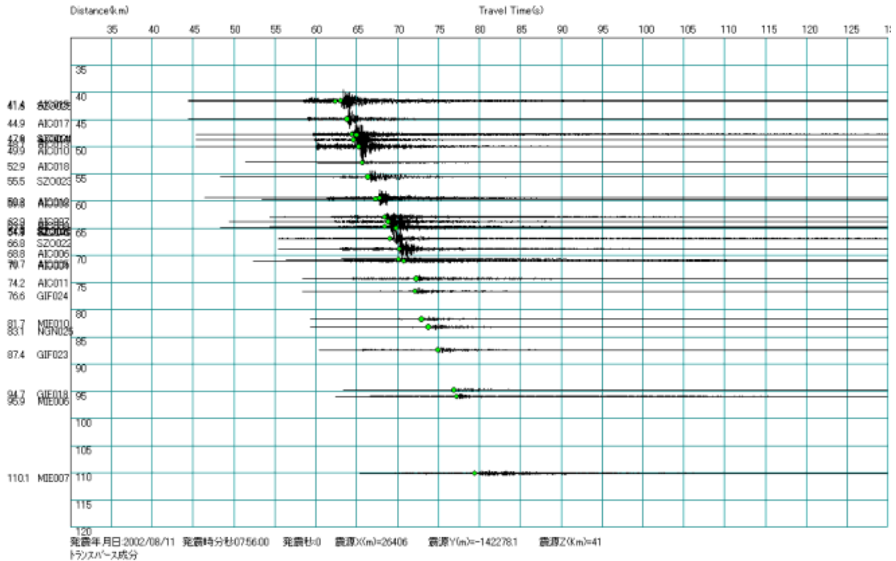
図 A1.1 トランスバースに変換した波形の一例 (2002 年 8 月 11 日 静岡県西部地震)
