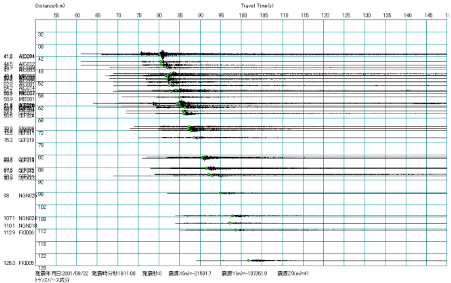
図 A1.4 トランスバースに変換した波形の一例 (2001 年 9 月 22 日 愛知県西部地震)
