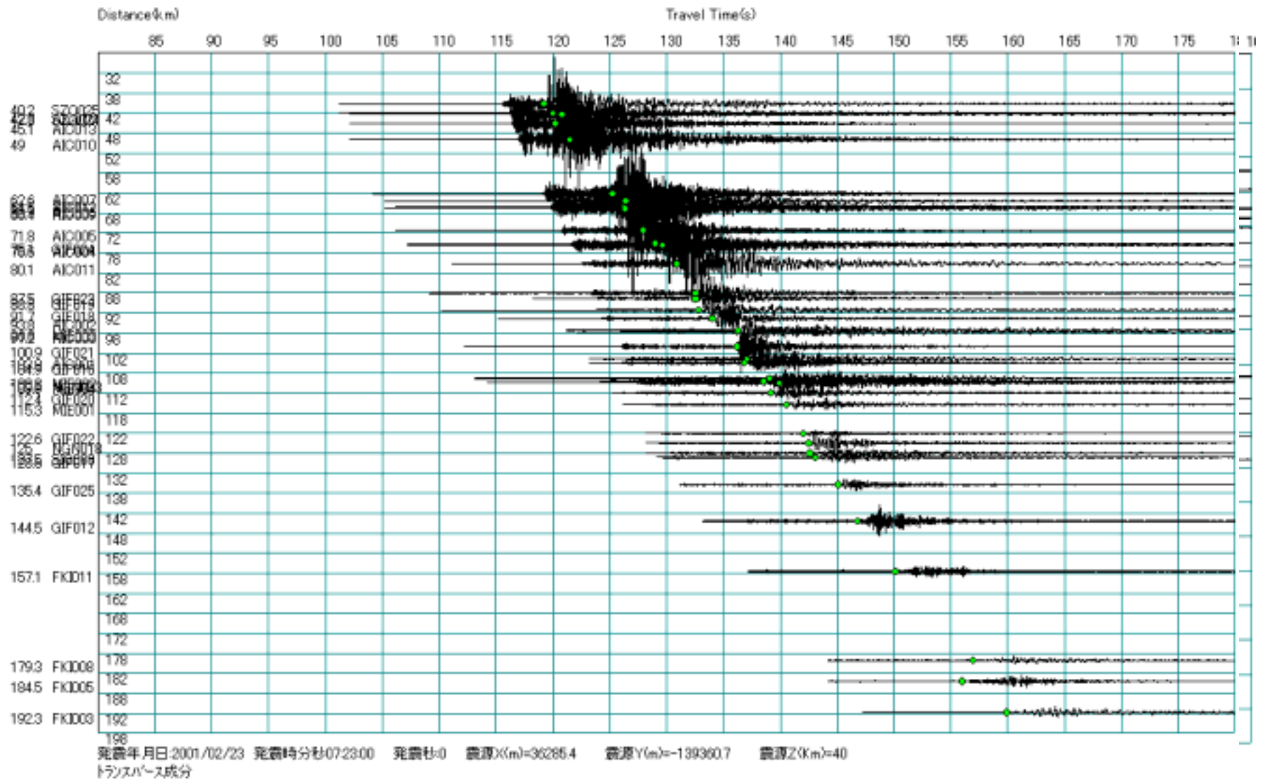
図 A1.12 トランスバースに変換した波形の一例（1998年12月2日 三重県北部地震）
