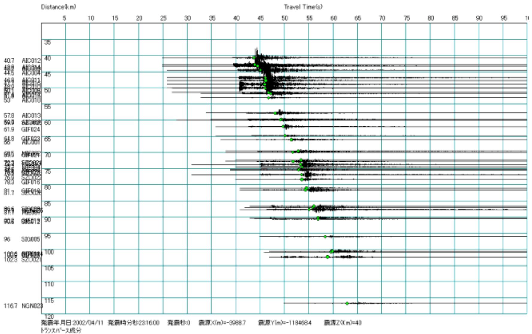
図 A1.2 トランスバースに変換した波形の一例 (2002 年 4 月 11 日 愛知県西部地震)
