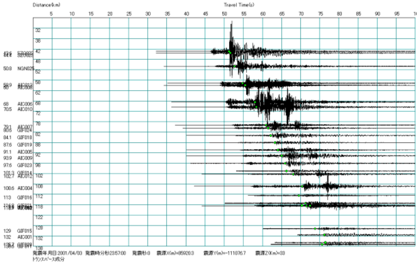
図 A1.5 トランスバースに変換した波形の一例 (2001年4月3日 静岡県中部地震)
