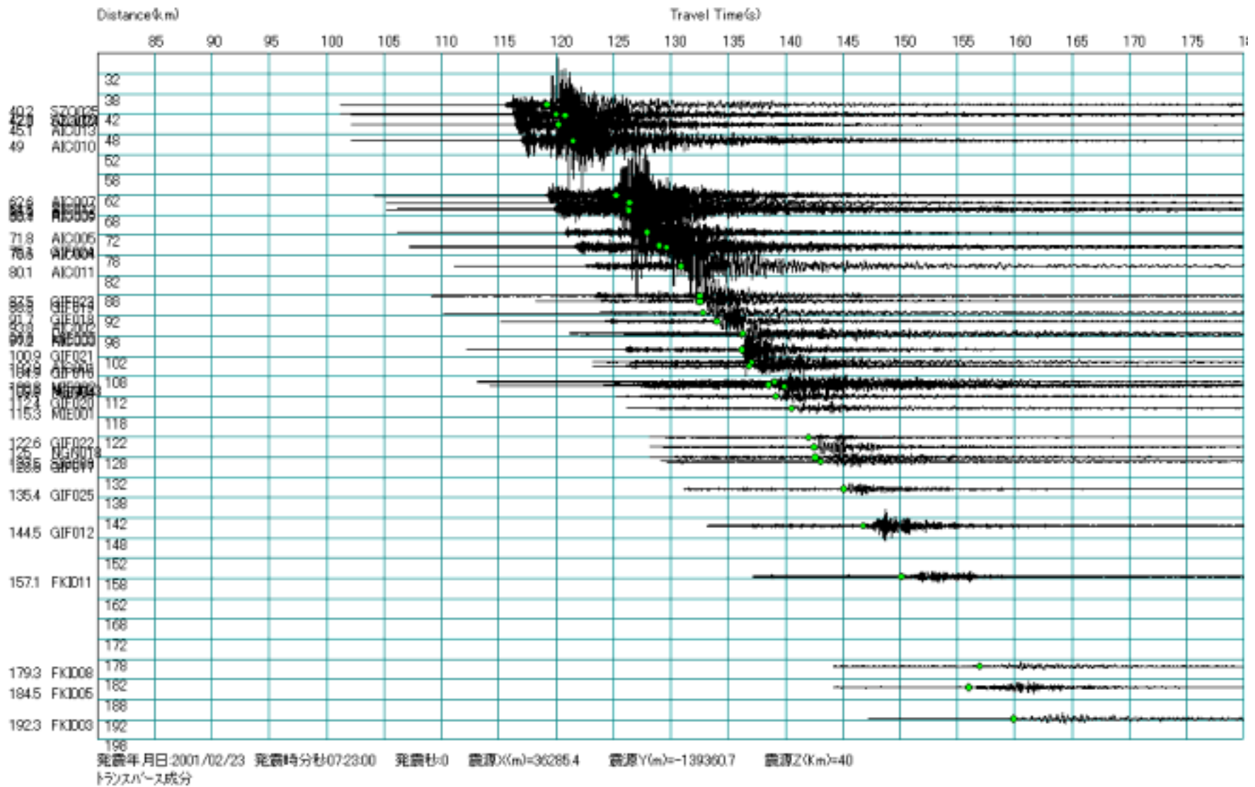
図 A1.11 トランスバースに変換した波形の一例 (1999 年 11 月 29 日 愛知県西部地震)
