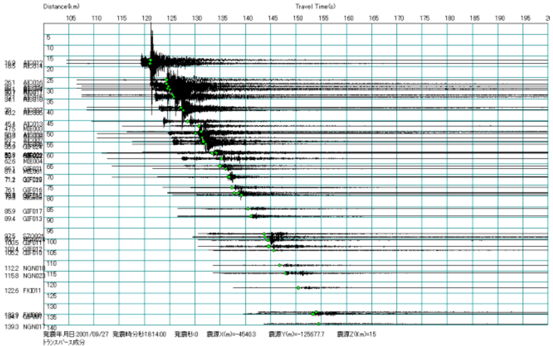
図 A1.3 トランスバースに変換した波形の一例 (2001 年 9 月 27 日 愛知県西部地震)
