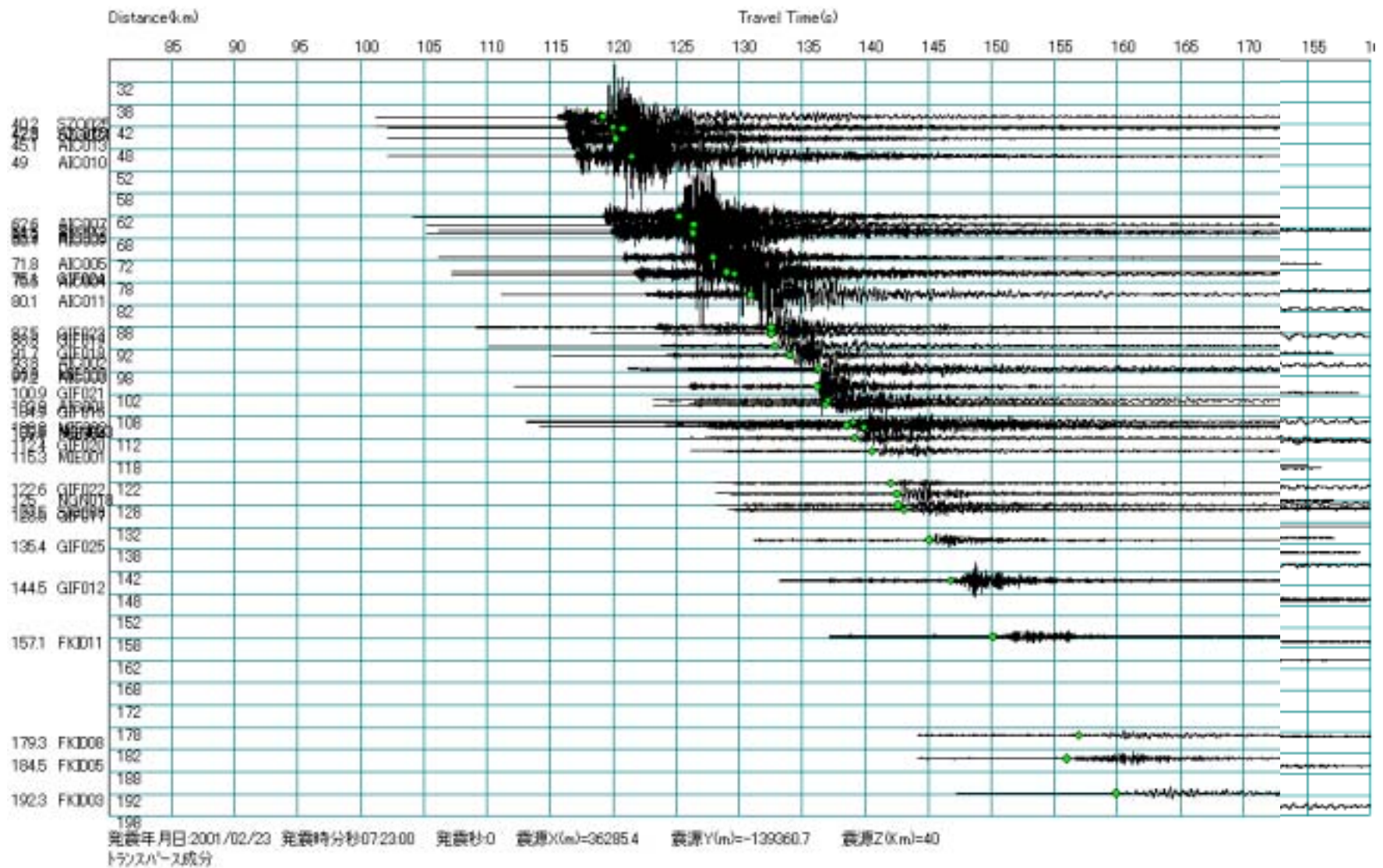
図 A1.16 トランスバースに変換した波形の一例 (1997年3月16日 愛知県東部地震)
