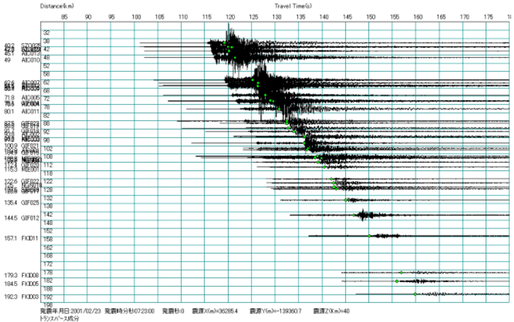
図 A1.7 トランスバースに変換した波形の一例（2001年1月6日 岐阜県美濃東部地震）
