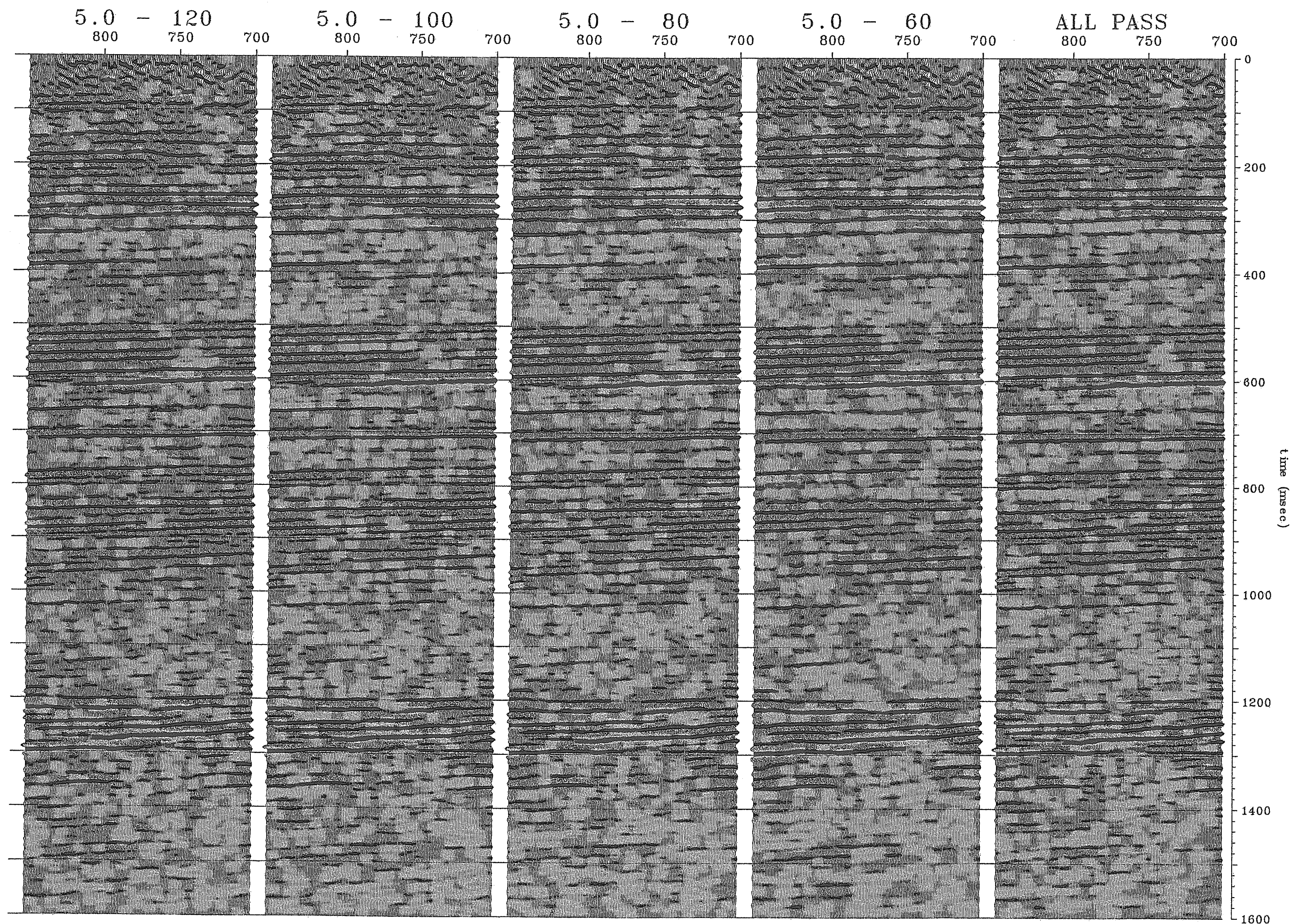
図 3. 1. 12 (1) ハイカットフィルターテスト (Line1 測線, CMP700~849)
