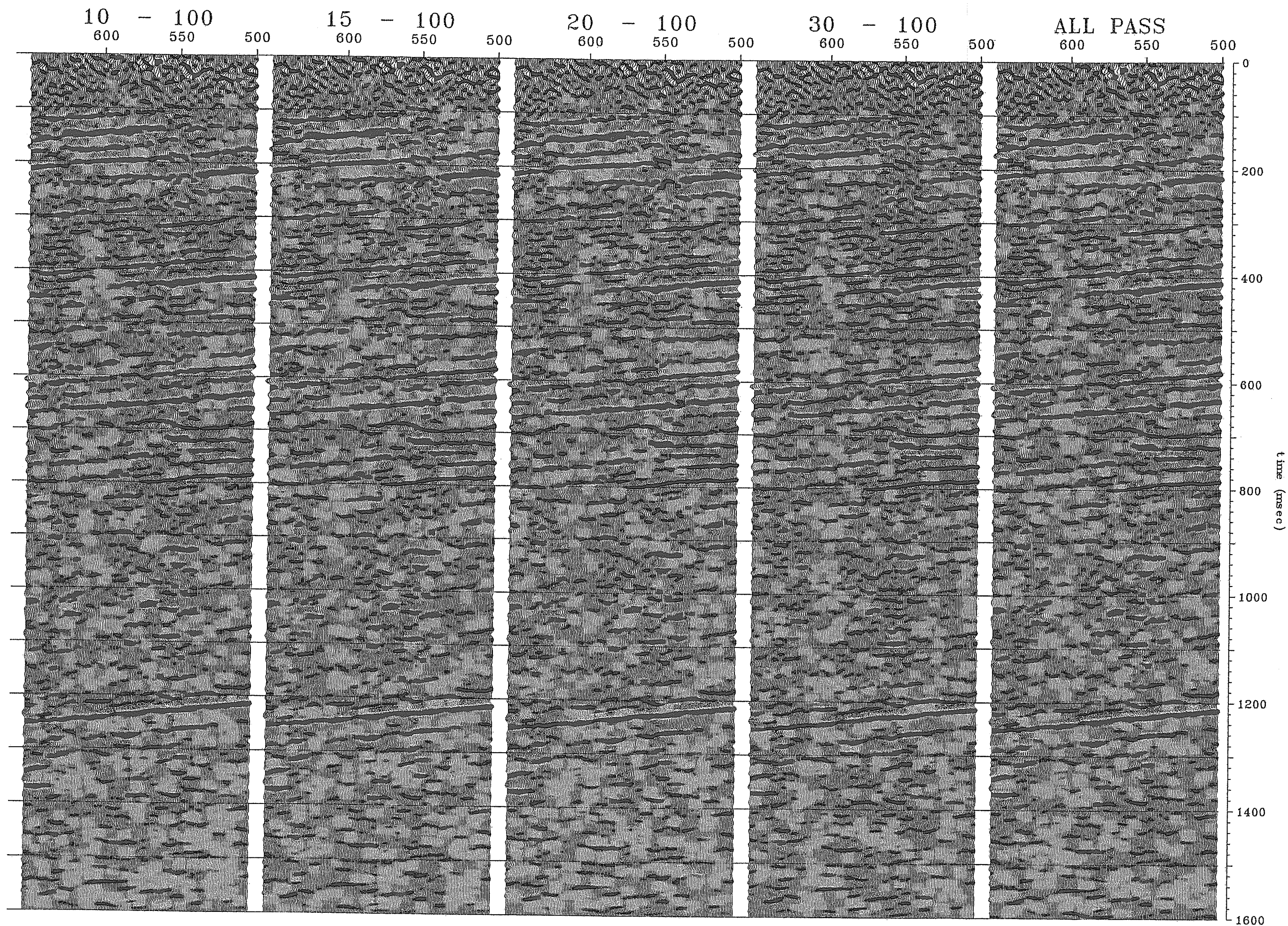
図 3. 1. 12 (4) ローカットフィルターテスト (Line2 測線, CMP500~649)
