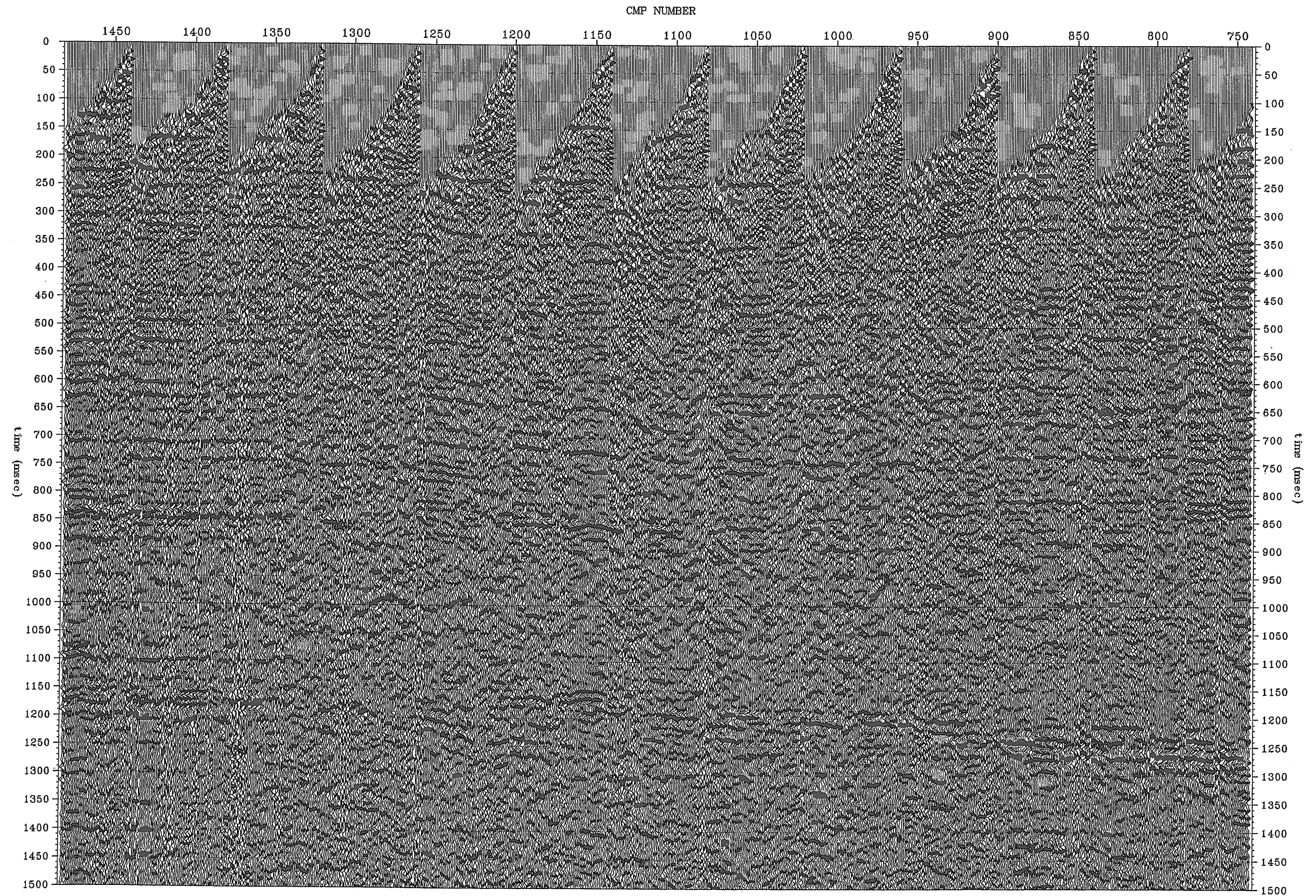
図 3. 1. 11 (6) -2 \tau - p フィルター後の 100% 断面 (Line2 測線, CMP741~1480)
