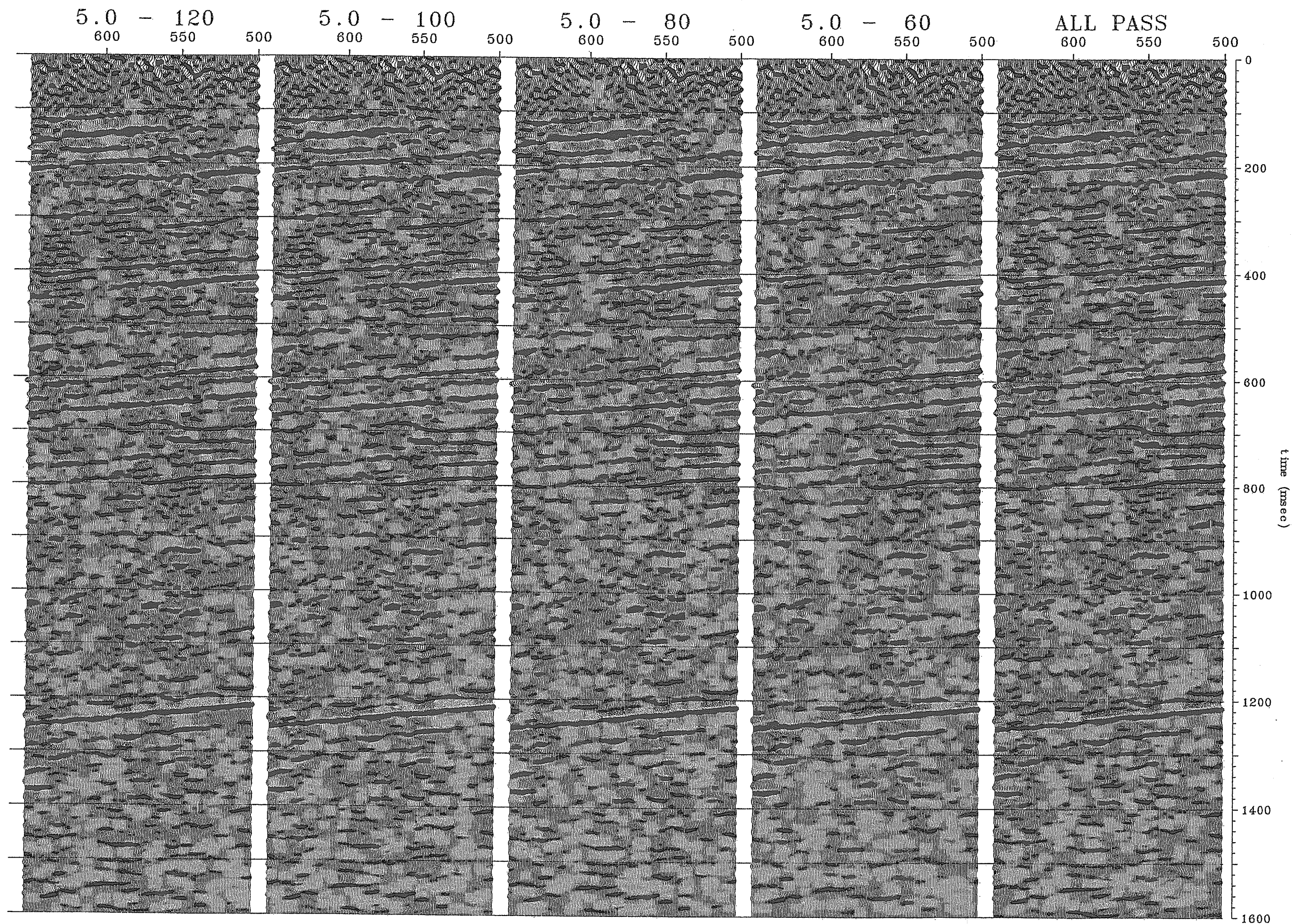
図 3. 1. 12 (3) ハイカットフィルターテスト (Line2 測線, CMP500~649)
