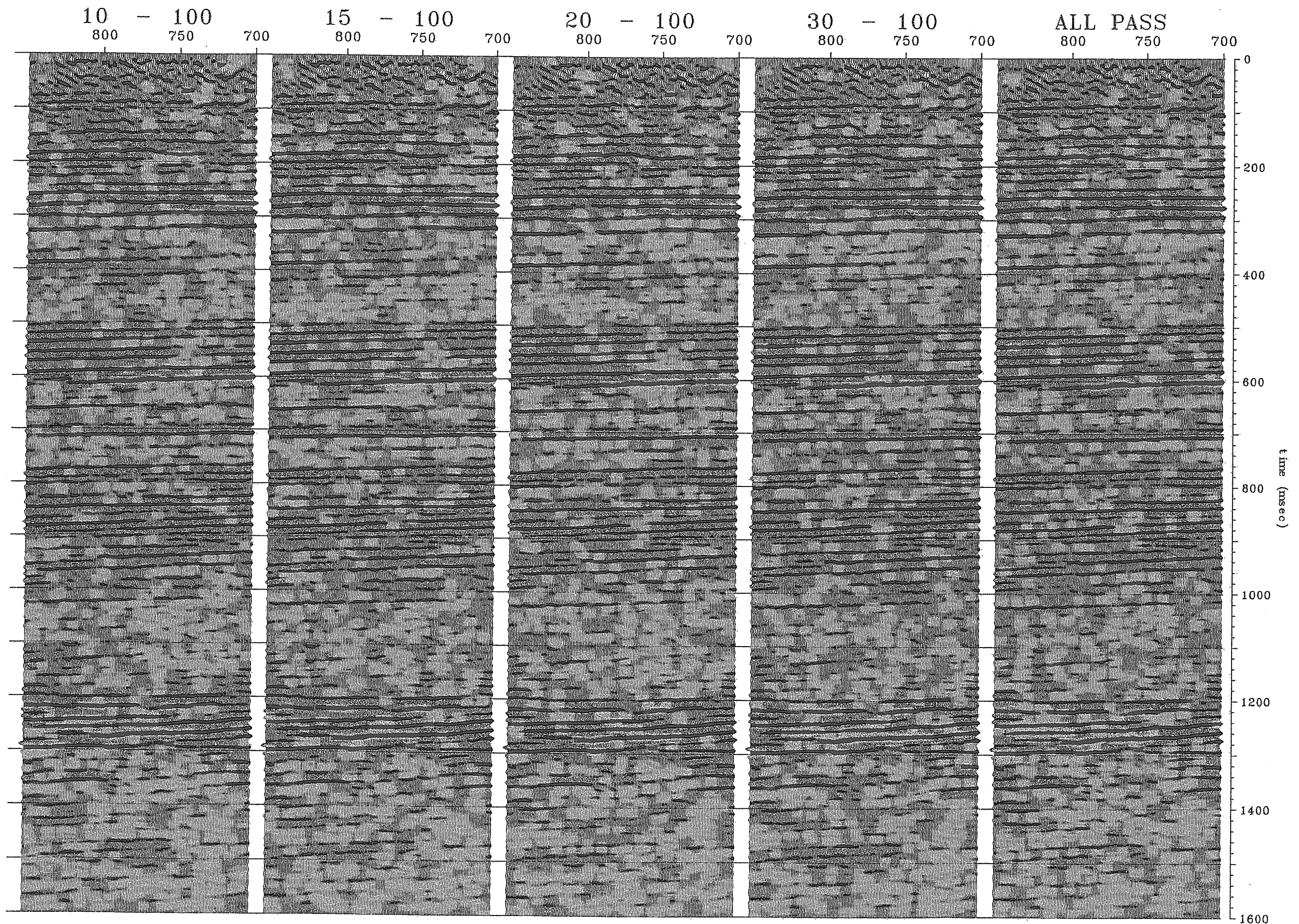
図 3. 1. 12 (2) ローカットフィルターテスト (Line1 測線, CMP700~849)
