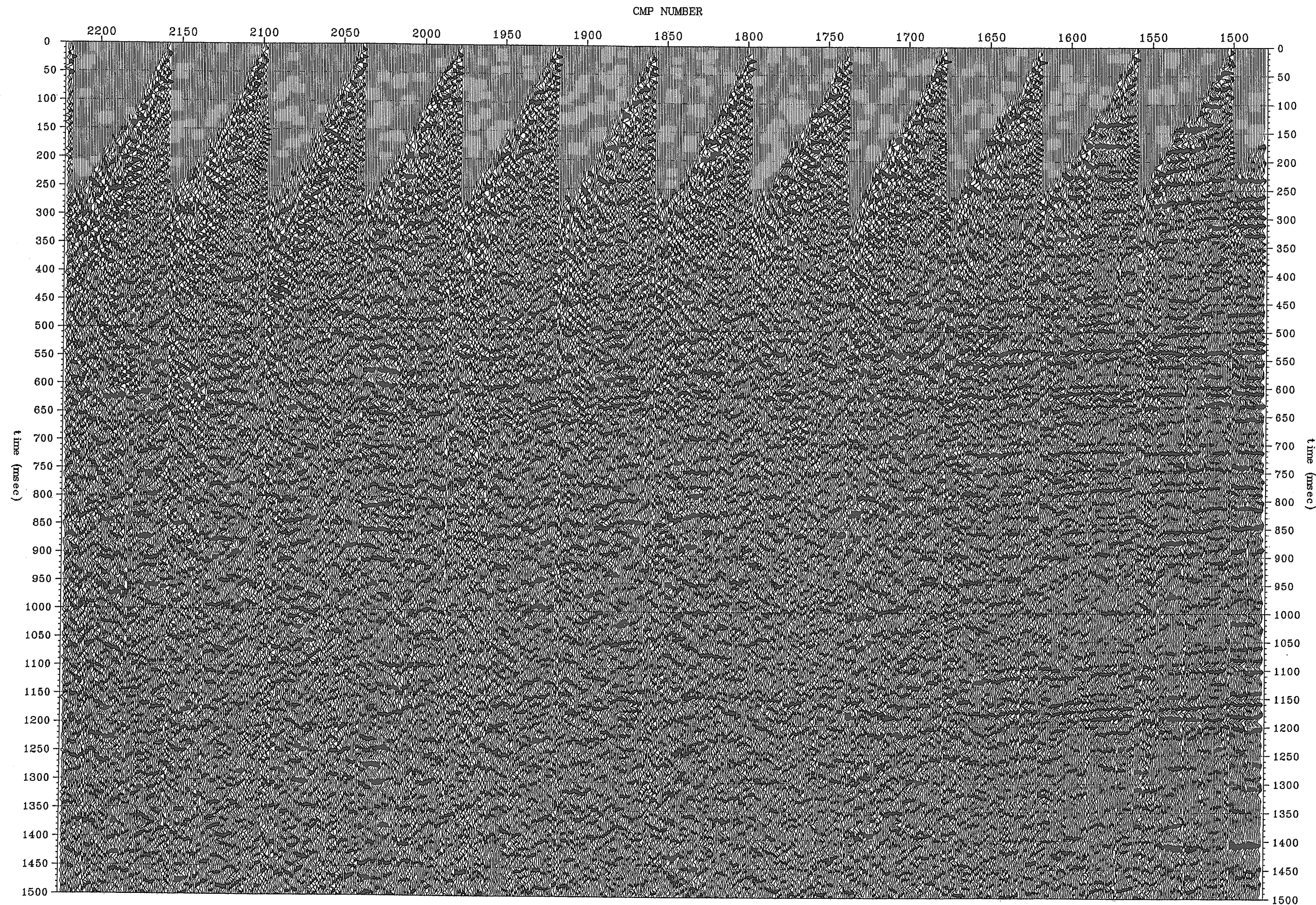
図 3. 1. 11 (6) -3 \tau - p フィルター後の 100%断面 (Line2 測線, CMP1481~2220)
