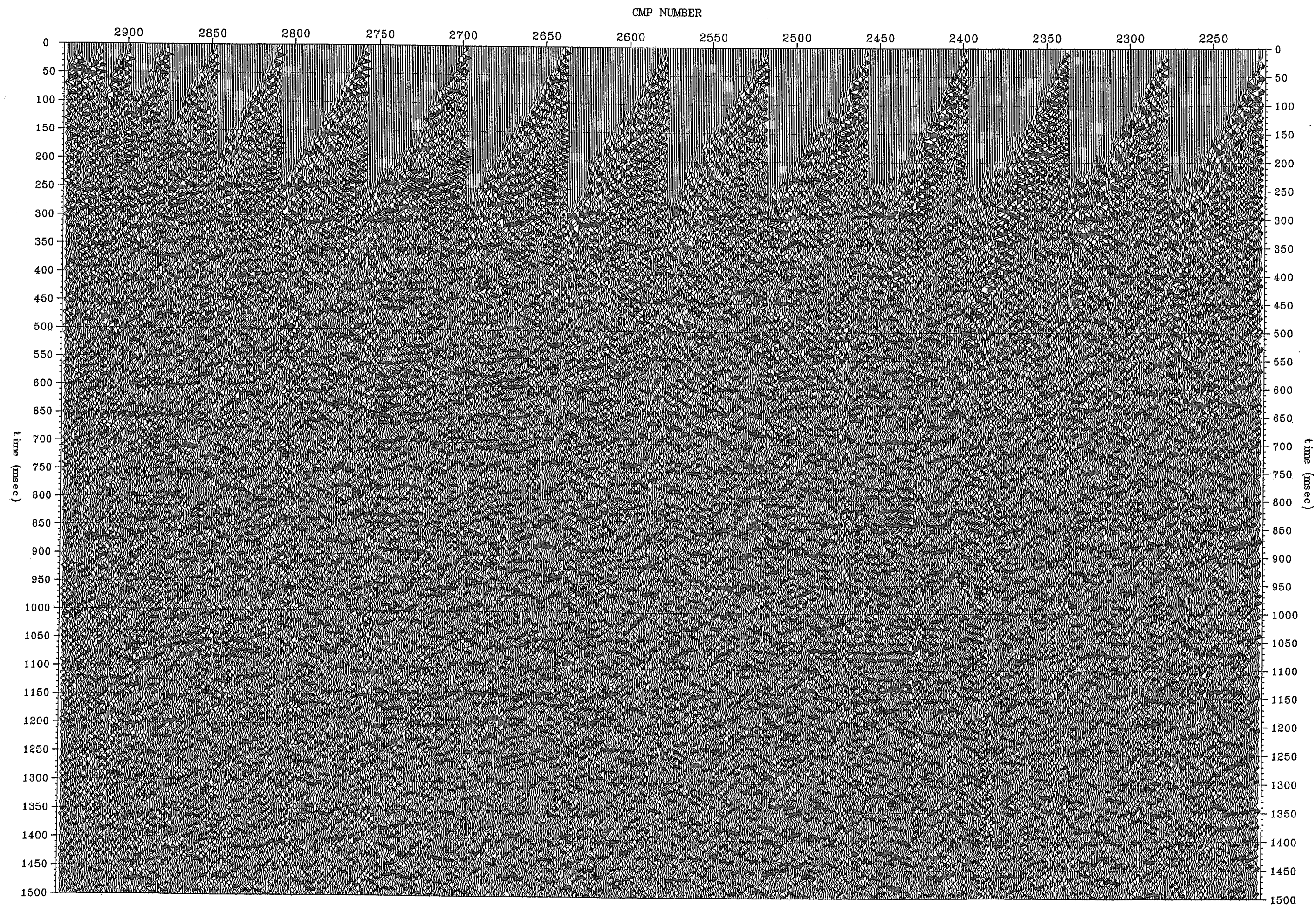
図 3. 1. 11 (6) -4 \tau - p フィルター後の 100%断面 (Line2 測線, CMP2221~2957)
