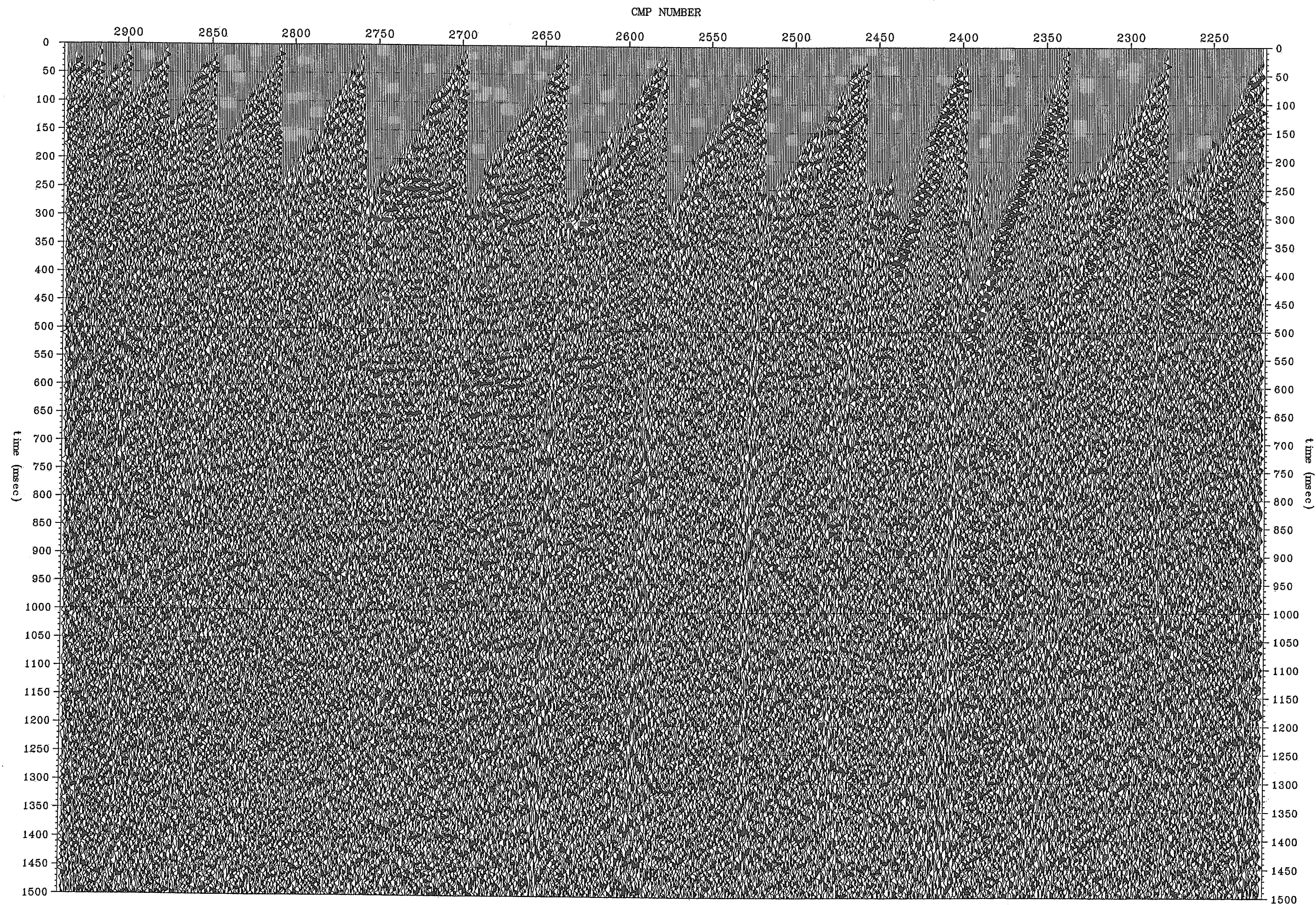
図 3. 1. 11 (5) -4 NMO補正後の100%断面 (Line2 測線, CMP2221~2957)
