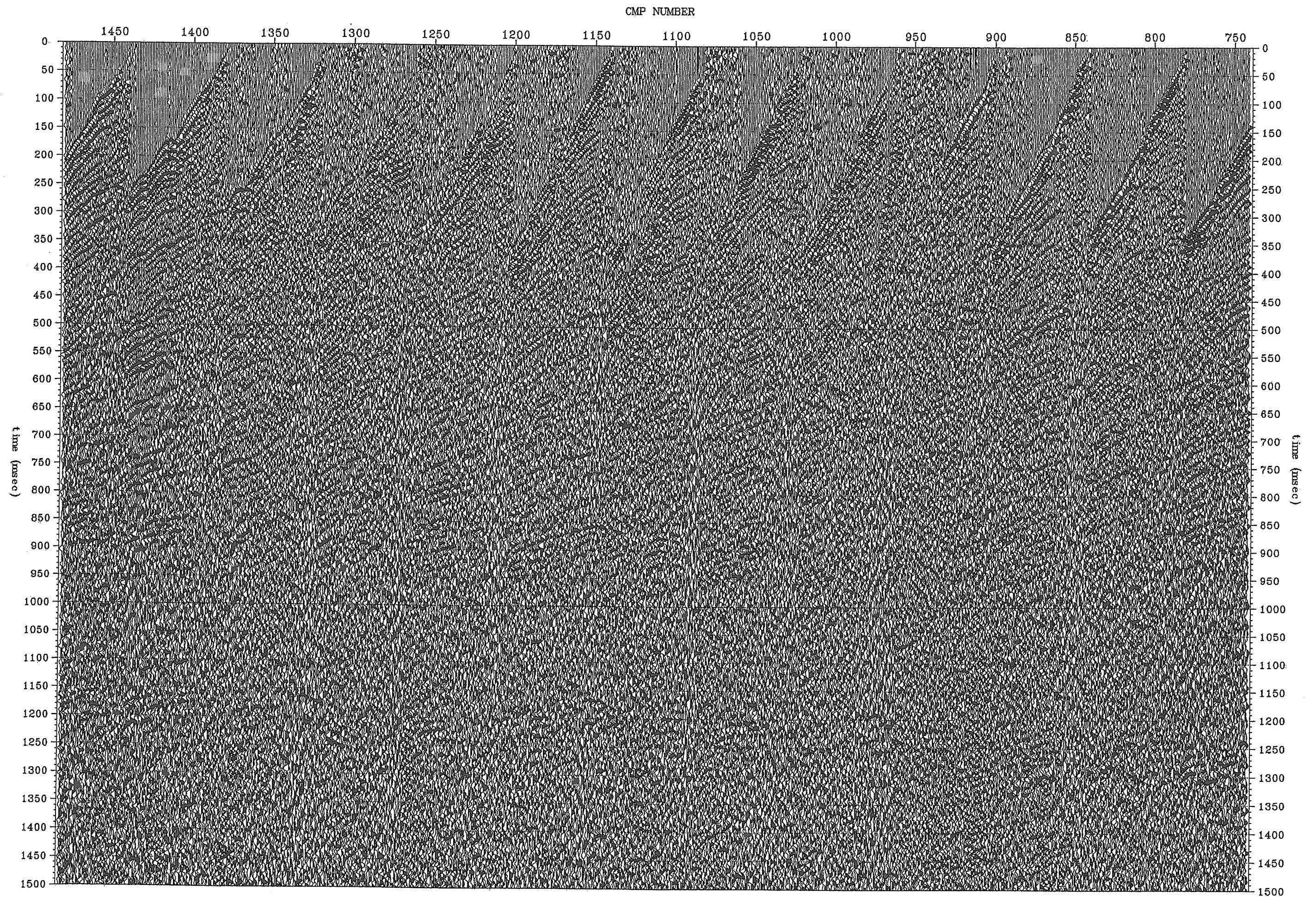
図 3. 1. 11 (3) -2 静補正後の 100%断面 (Line2 測線, CMP741~1480)
