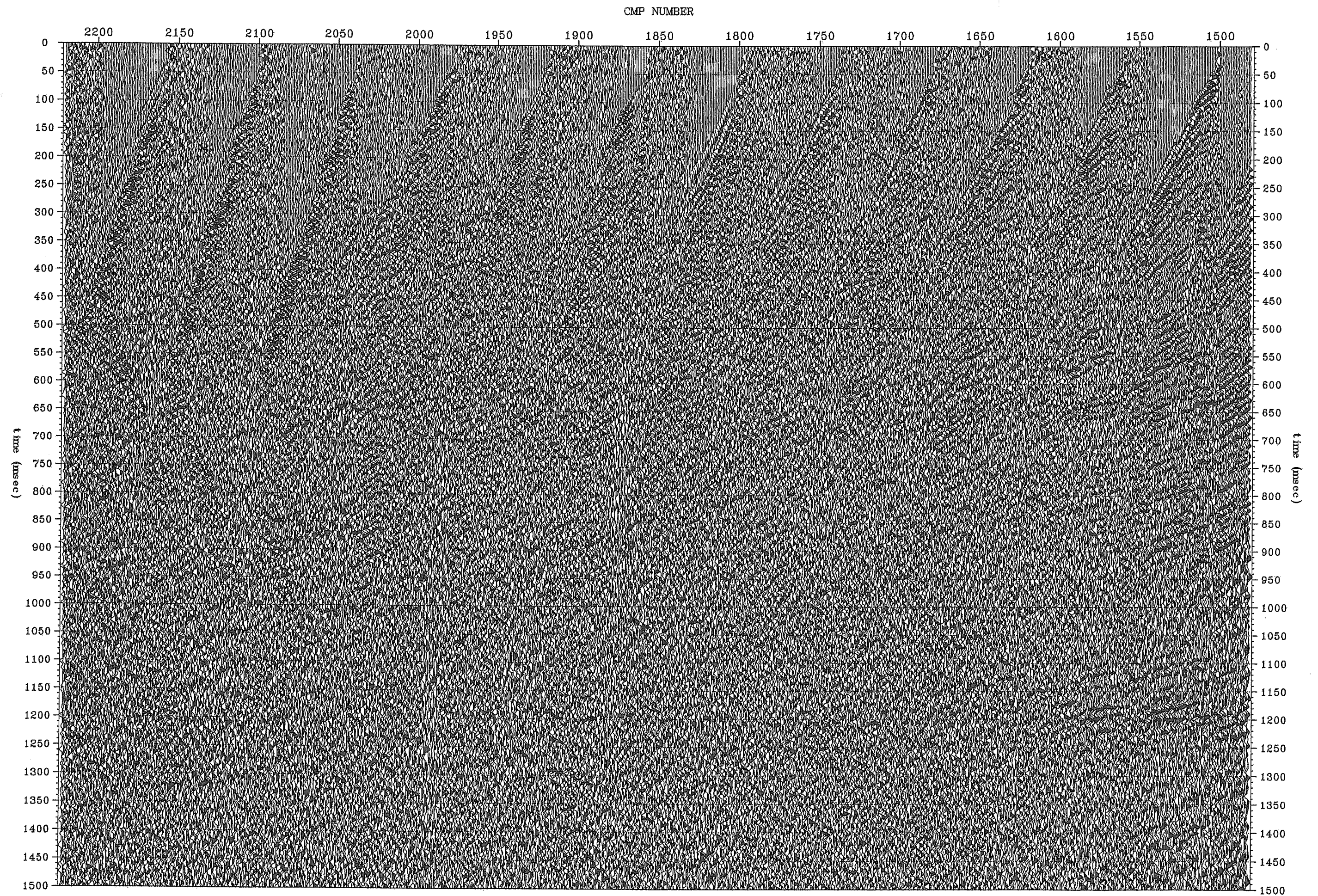
図 3. 1. 11 (4) -3 デコンボリューション後の 100%断面 (Line2 測線, CMP1481~2220)
