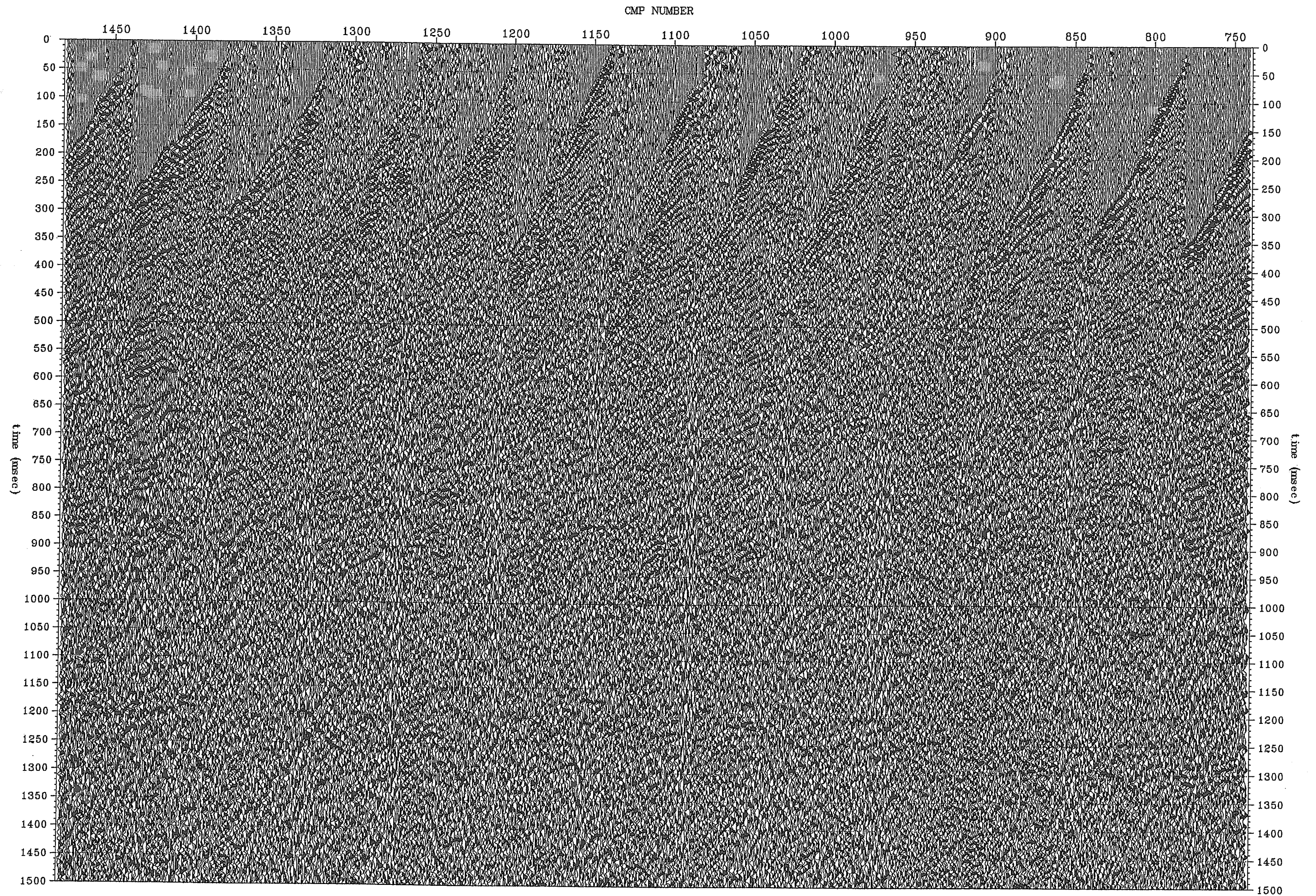
図 3. 1. 11 (4) -2 デコンボリューション後の 100%断面 (Line2 測線, CMP741~1480)
