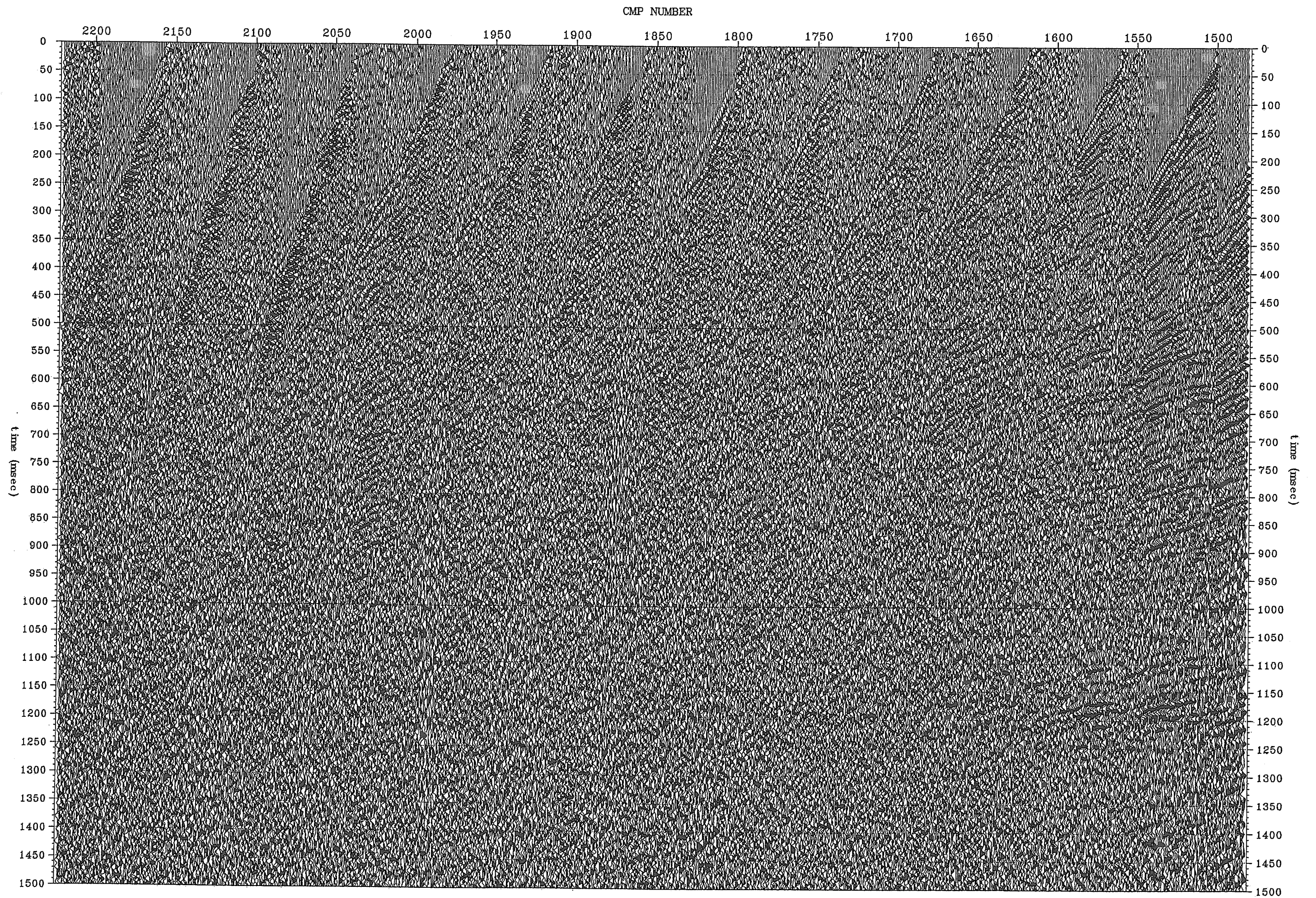
図 3. 1. 11 (3) -3 静補正後の 100%断面 (Line2 測線, CMP1481~2220)
