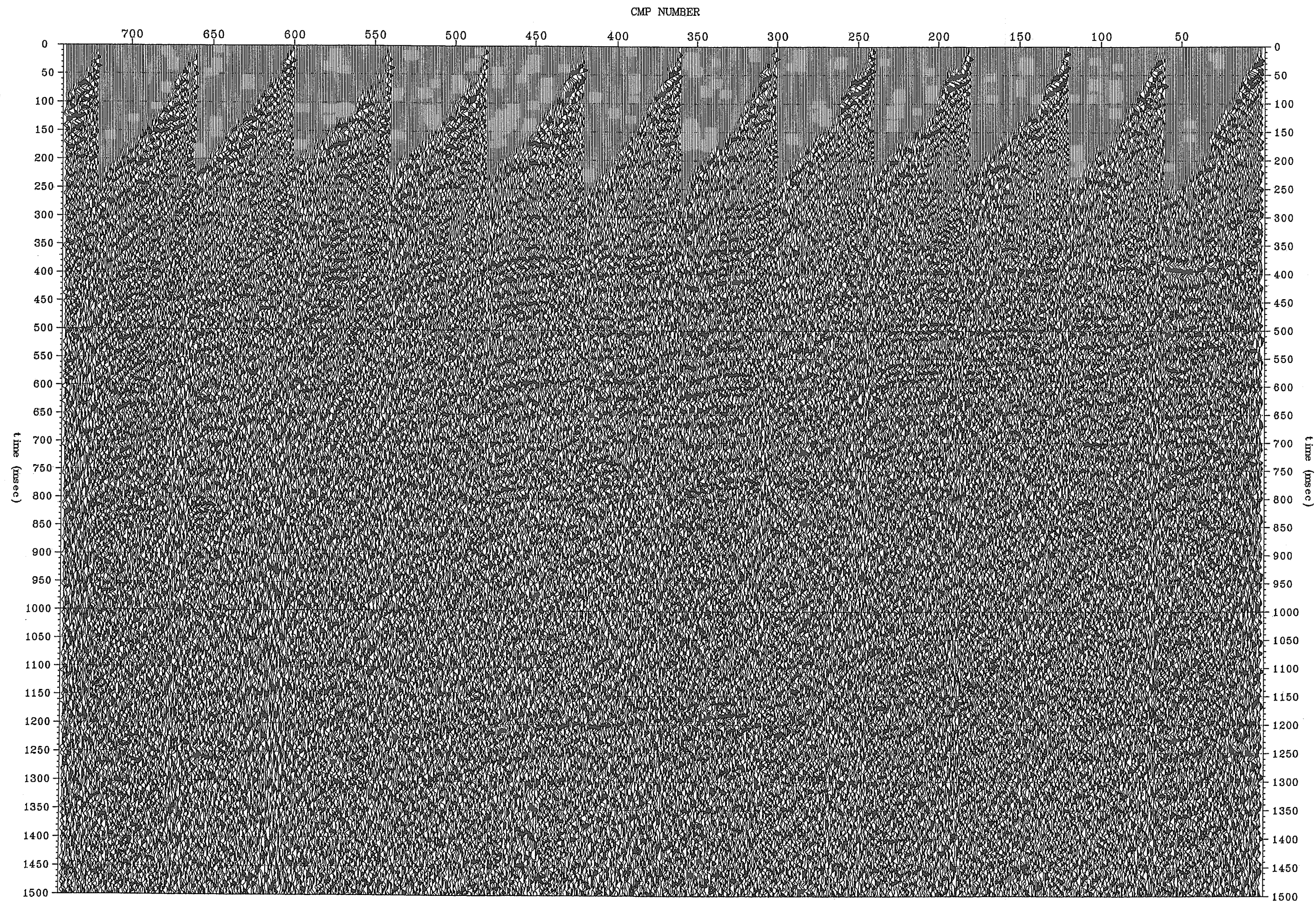
図 3.1.11 (5) -1 NMO補正後の 100%断面 (Line2 測線, CMP1~740)
