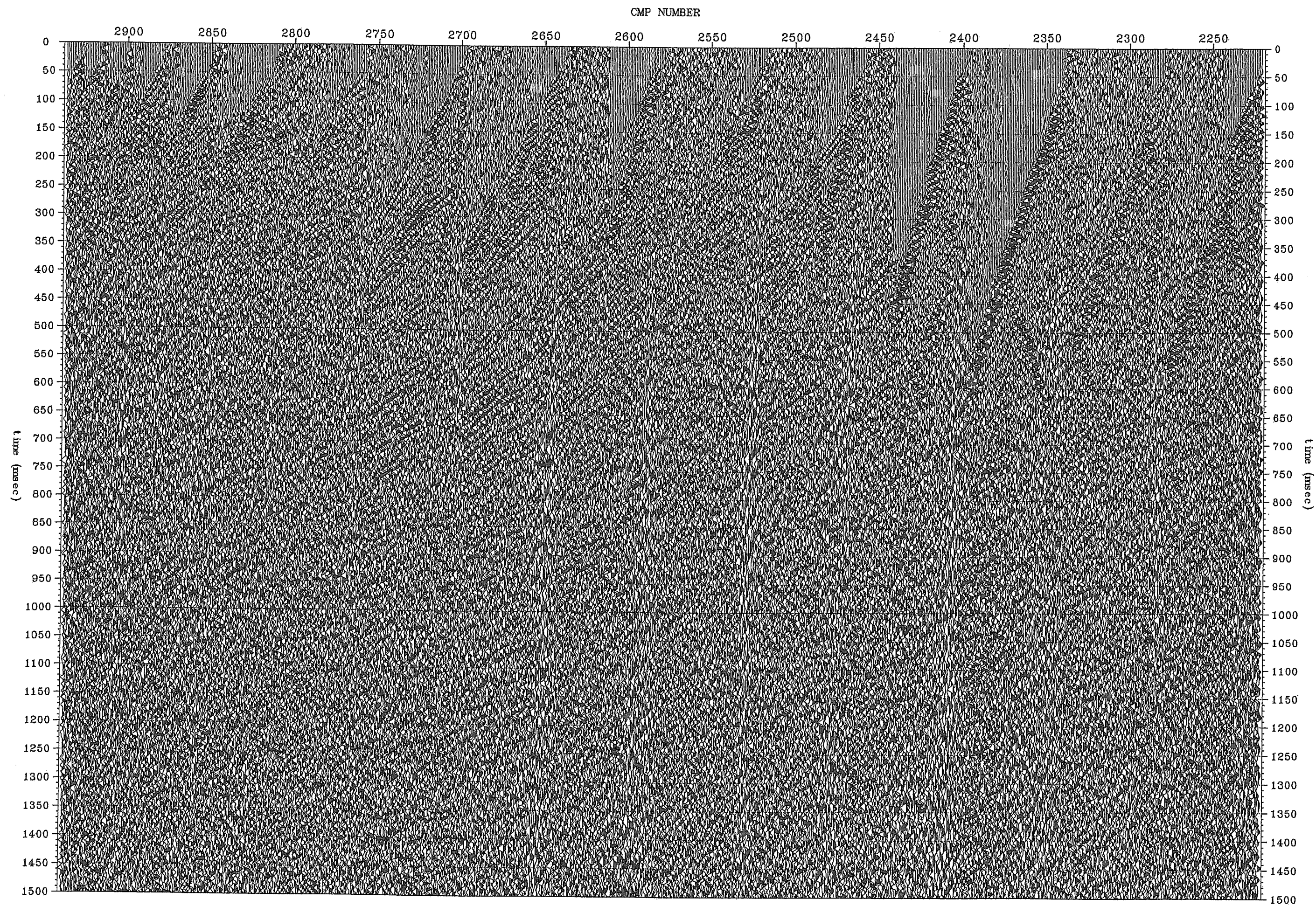
図 3. 1. 11 (3) -4 静補正後の 100%断面 (Line2 測線, CMP2221~2957)
