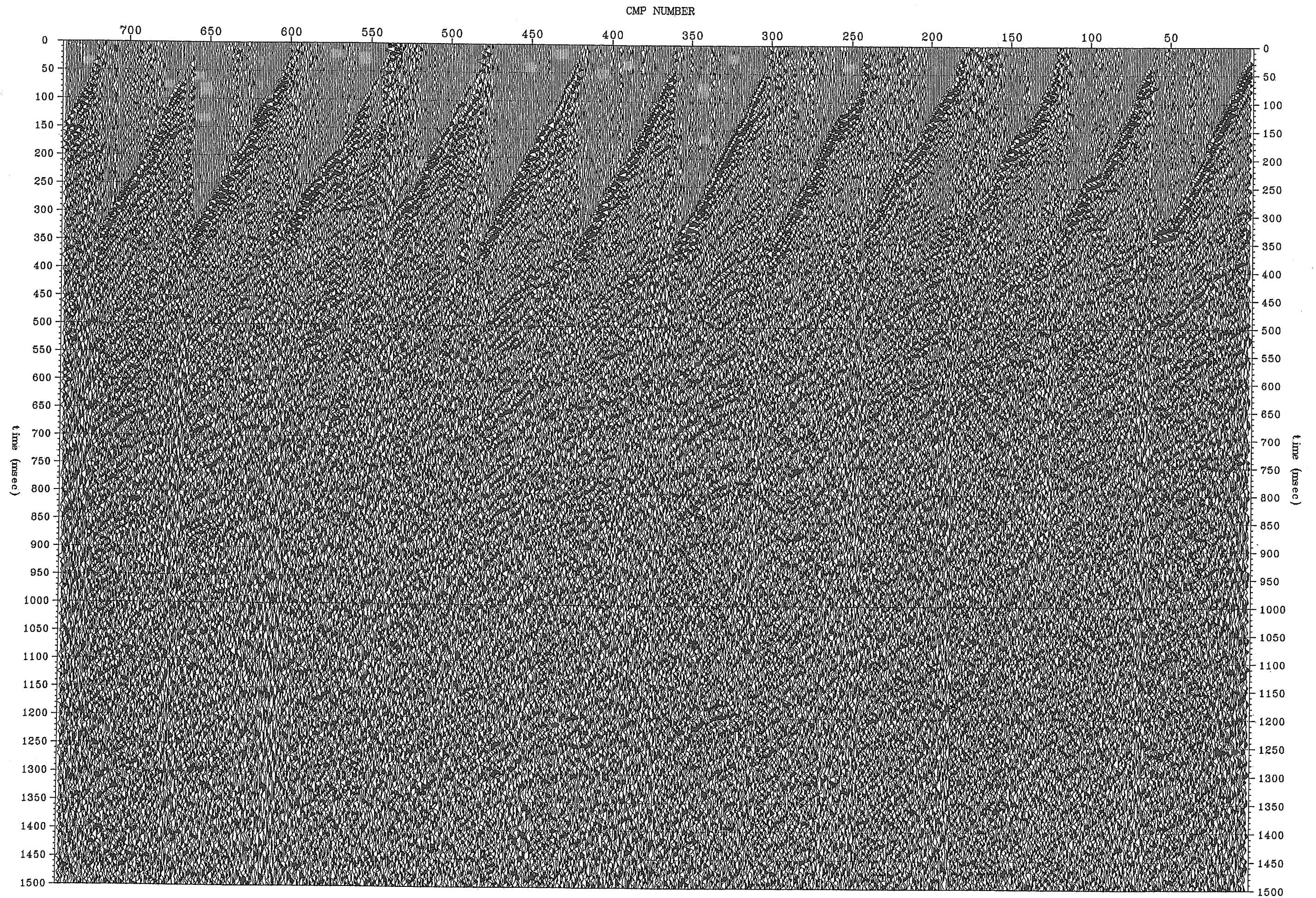
図 3. 1. 11 (4) -1 デコンボリューション後の 100%断面 (Line2 測線, CMP1~740)
