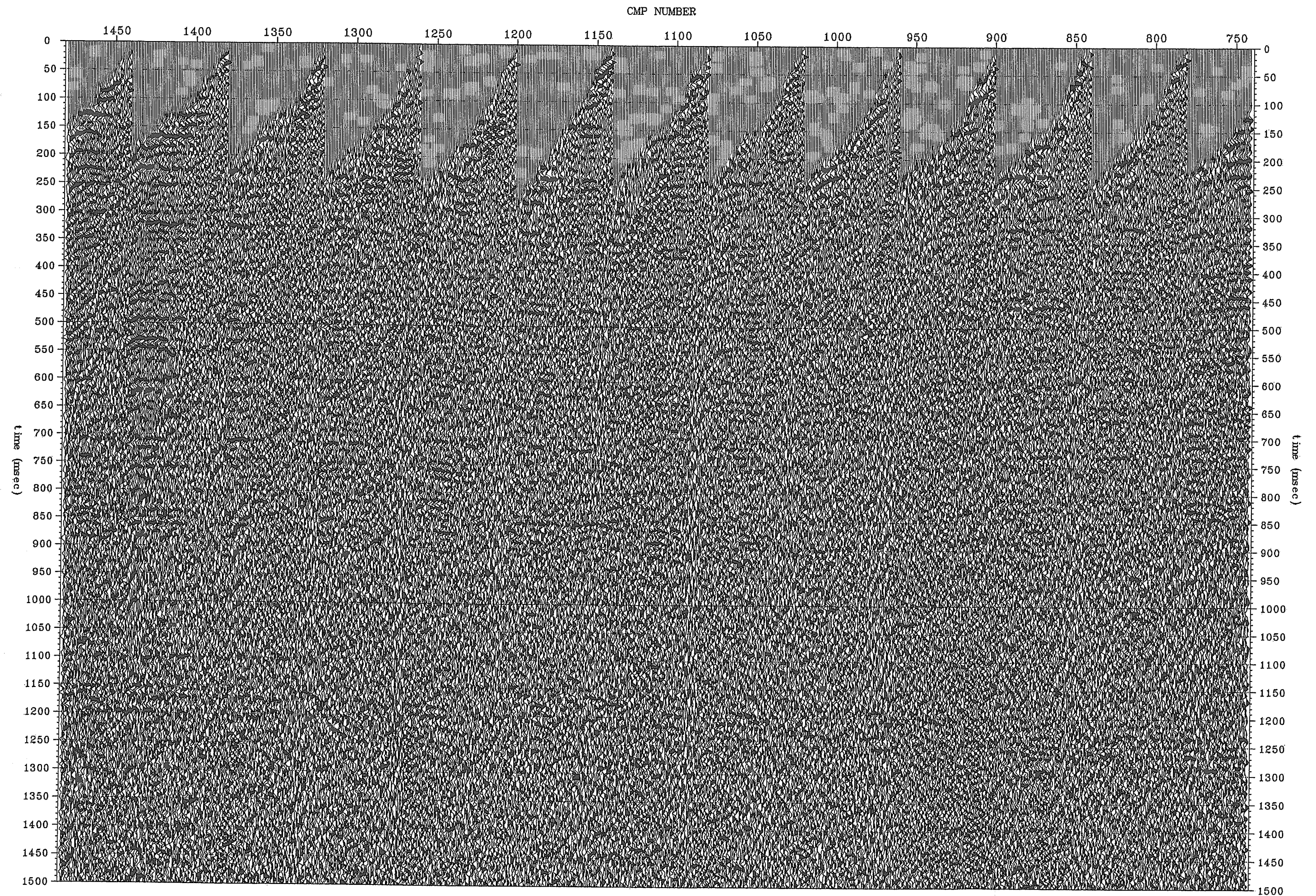
図 3. 1. 11 (5) -2 NMO補正後の 100%断面 (Line2 測線, CMP741~1480)
