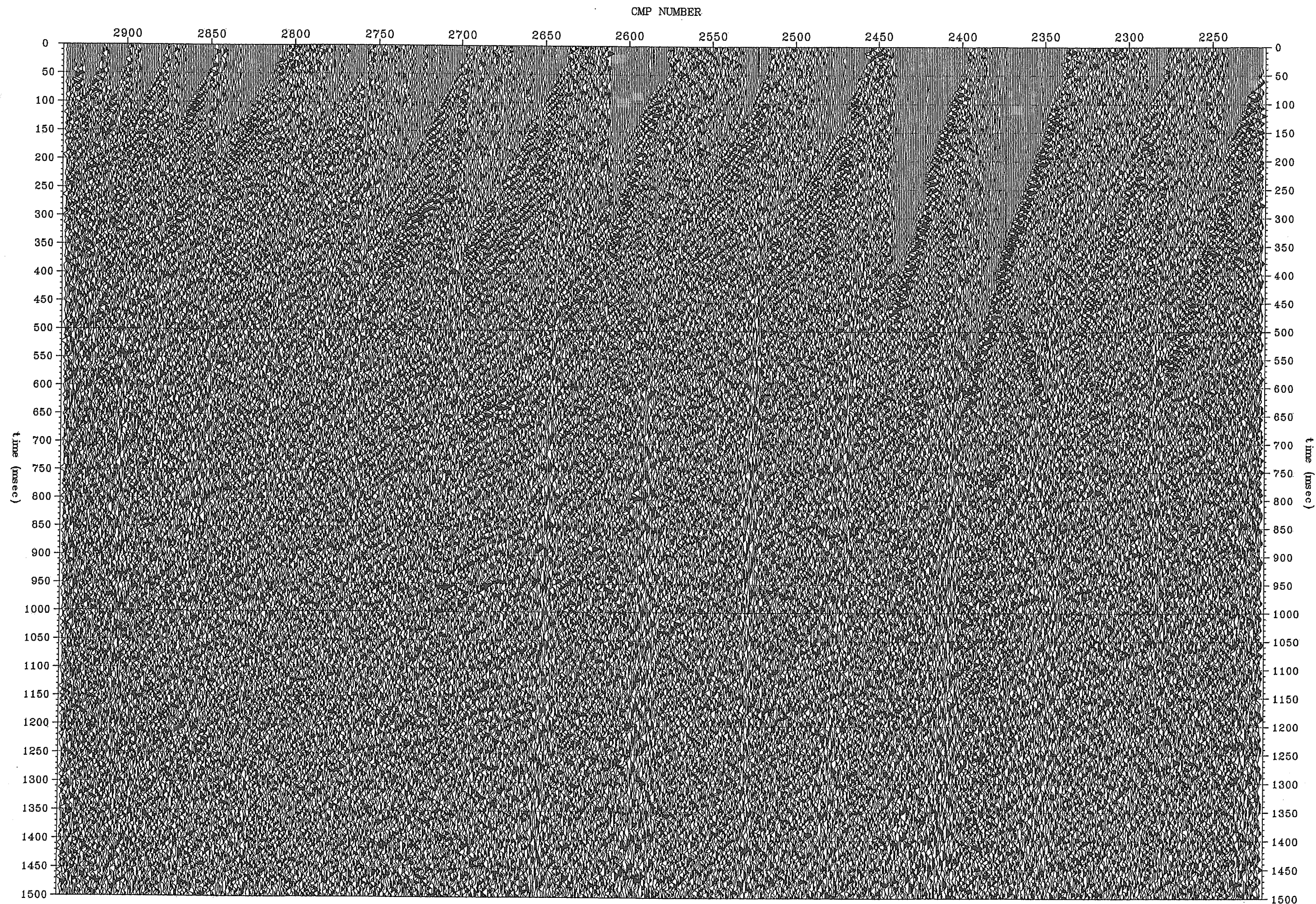
図 3. 1. 11 (4) -4 デコンボリューション後の 100%断面 (Line2 測線, CMP2221~2957)
