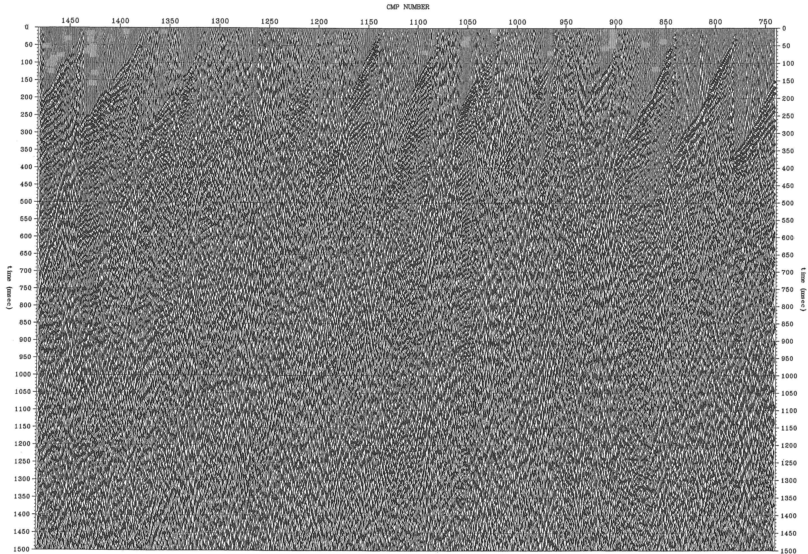
図 3. 1. 11 (2) -2 プレフィルタリング・位相補償・振幅調整後の 100%断面 (Line2 測線, CMP741~1480)
