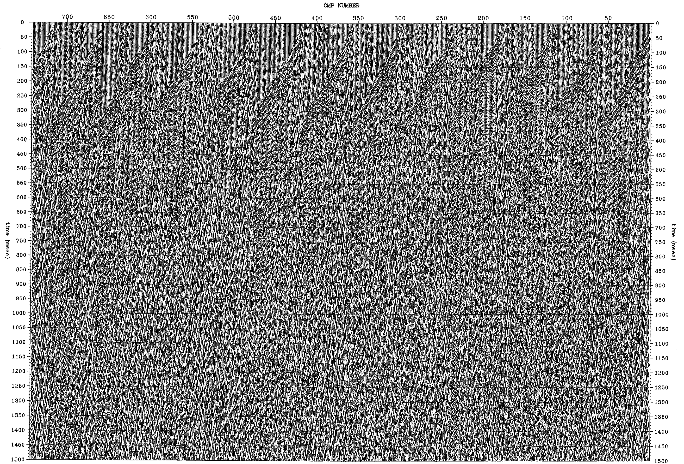
図 3. 1. 11 (2) -1 プレフィルタリング・位相補償・振幅調整後の 100%断面 (Line2 測線, CMP1~740)
