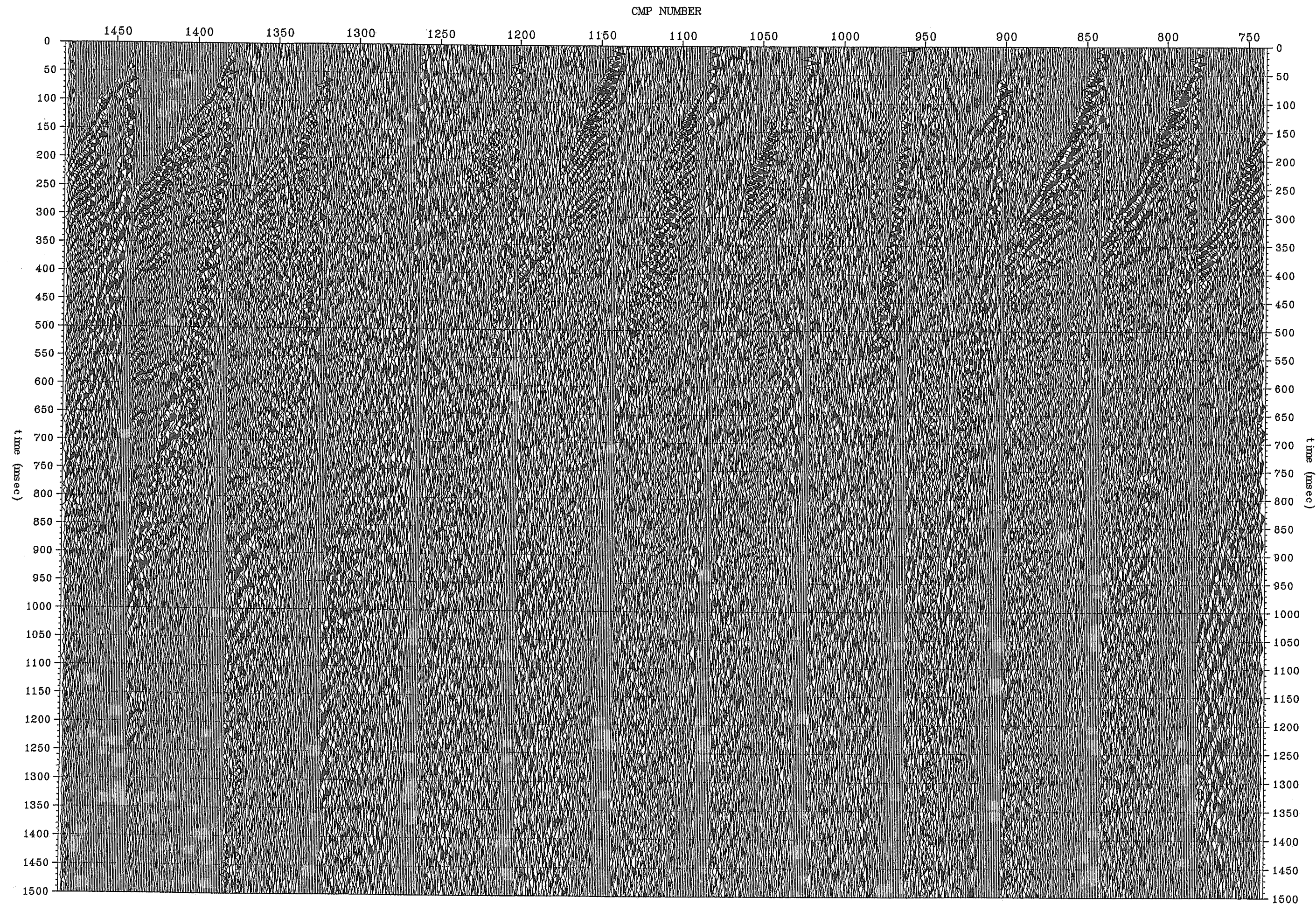
図 3. 1. 11 (1) -2 生波形の 100%断面 (Line2 測線, CMP741~1480)
