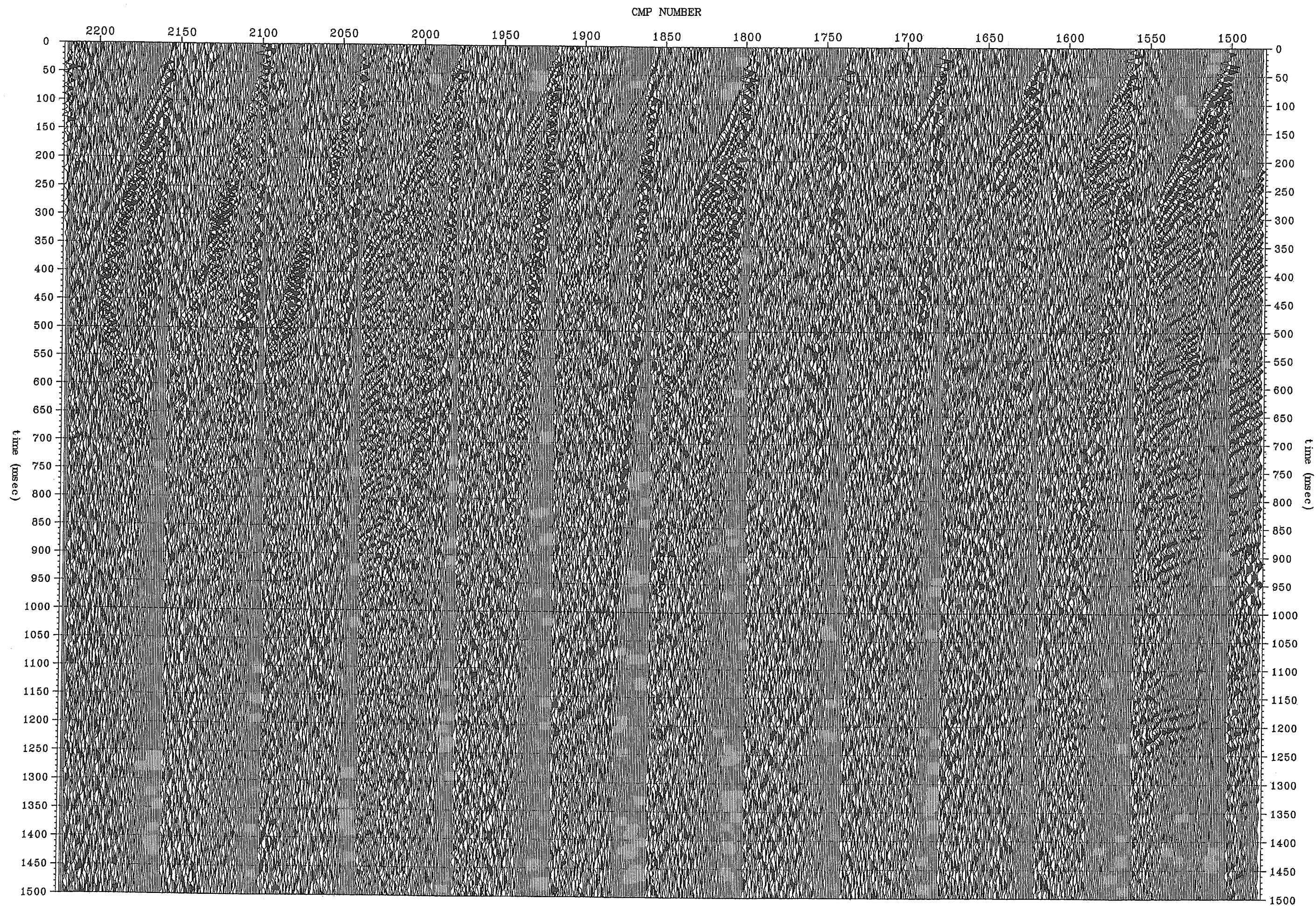
図 3.1.11 (1)-3 生波形の 100%断面 (Line2 測線, CMP1481~2220)
