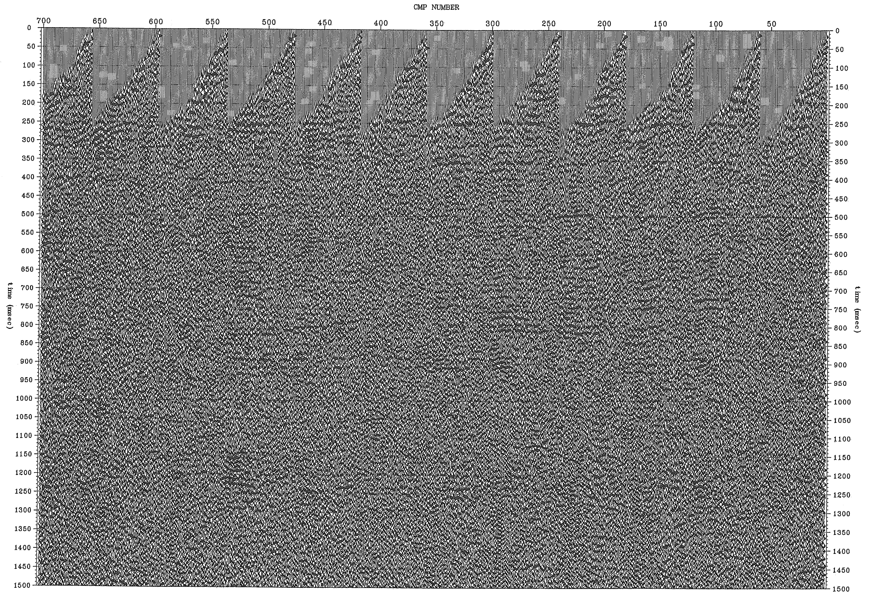
図 3. 1. 10 (6) -1 \tau - p フィルター後の 100%断面 (Line1 測線, CMP1~700)
