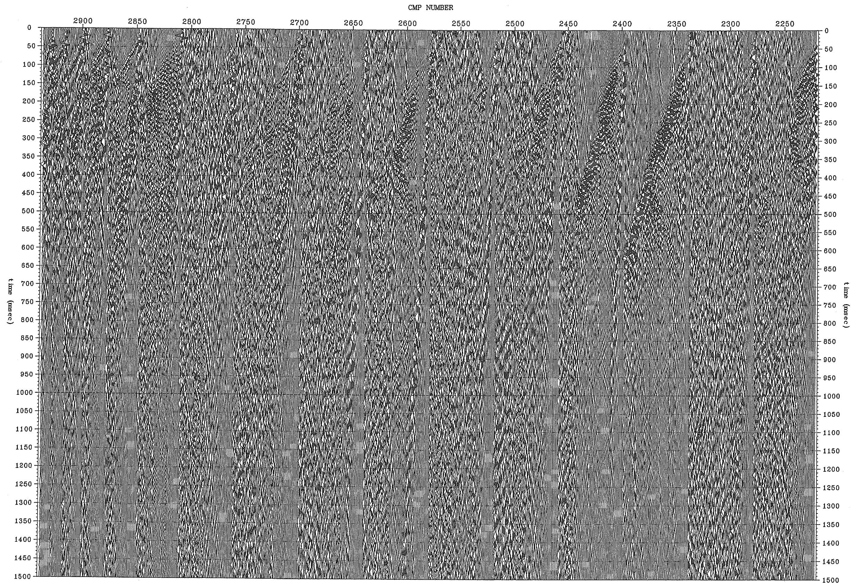
図 3.1.11 (1)-4 生波形の 100%断面 (Line2 測線, CMP2221~2957)
