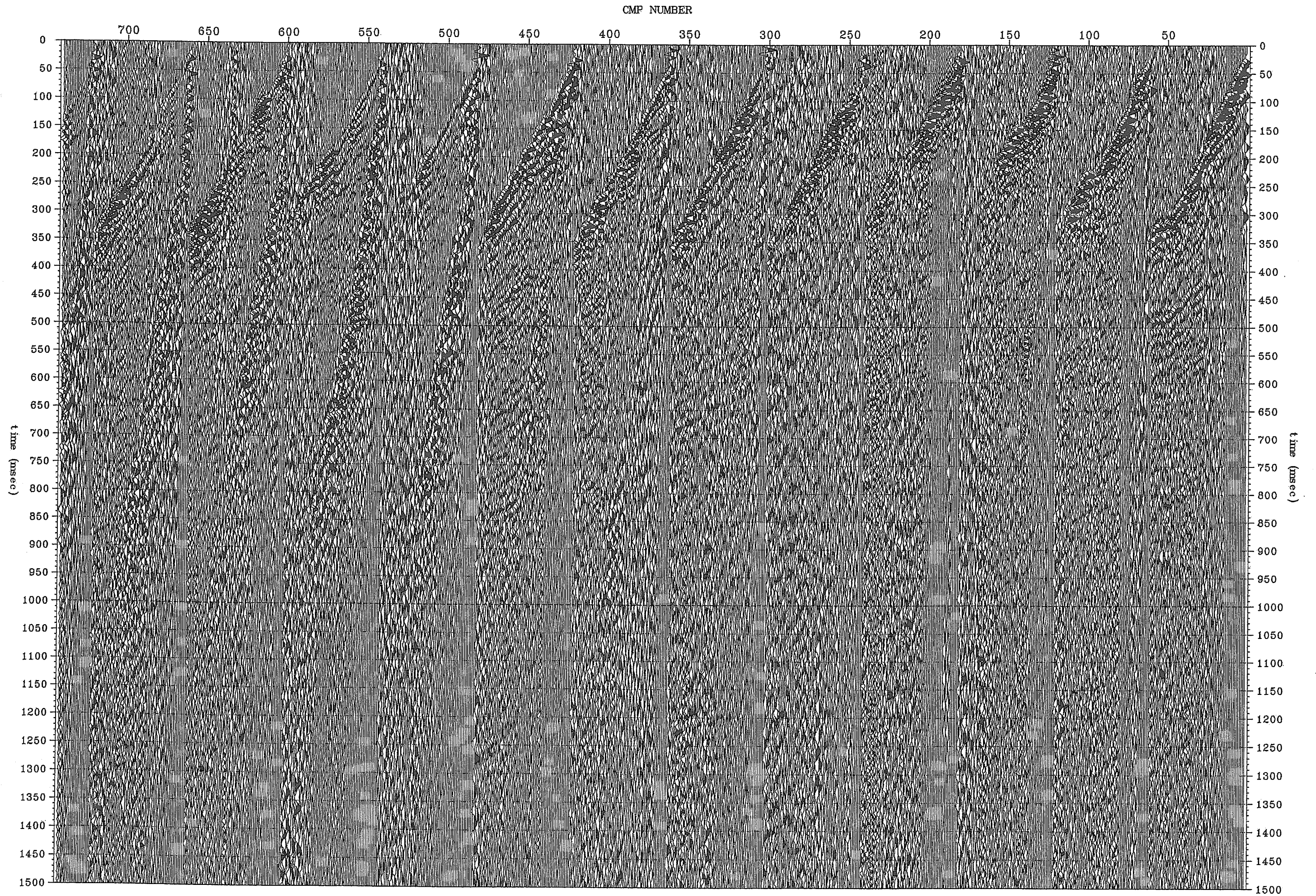
図 3. 1. 11 (1) -1 生波形の 100%断面 (Line2 測線, CMP1~740)
