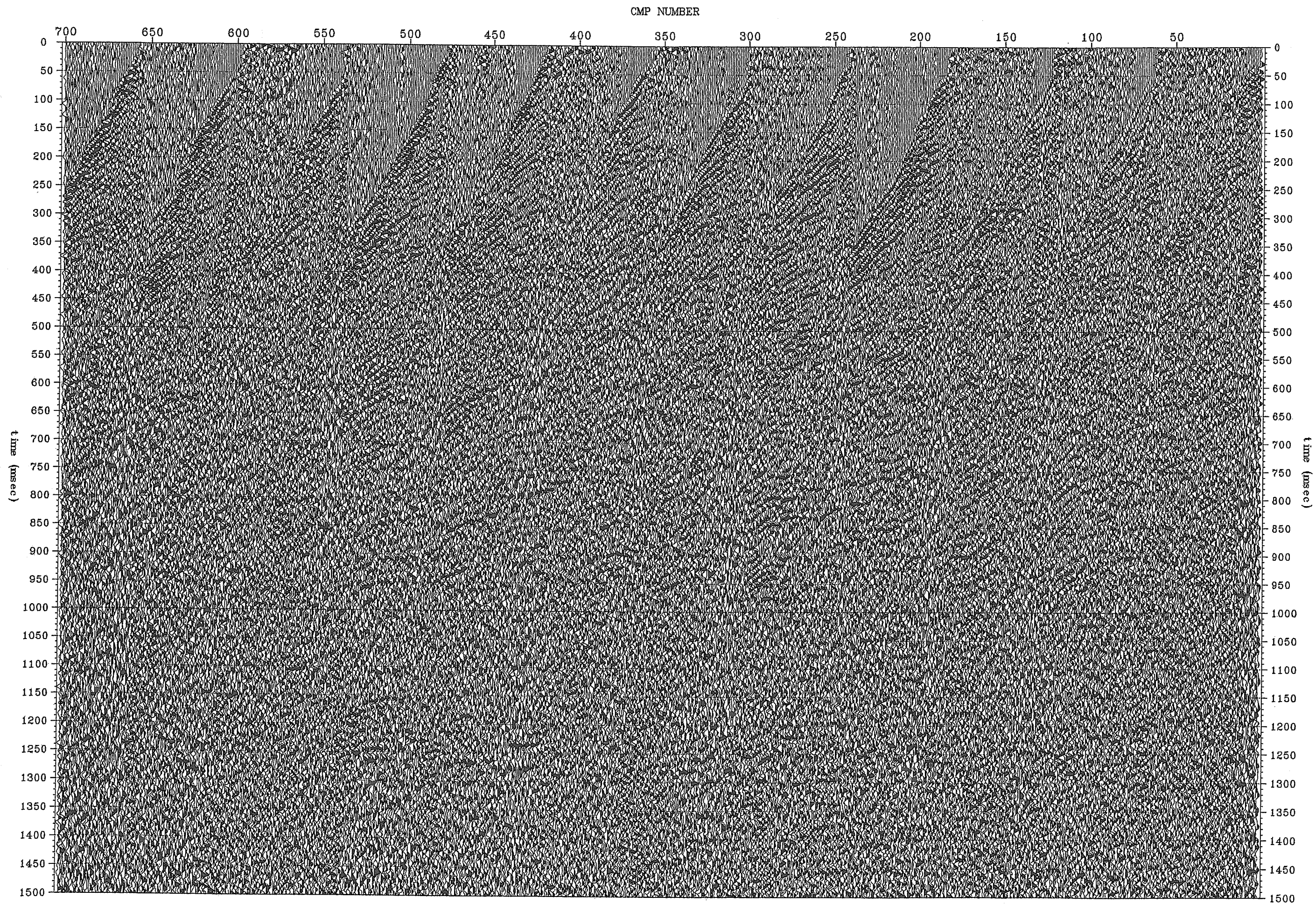
図 3.1.10 (4) -1 デコンボリューション後の 100%断面 (Line1 測線, CMP1~700)
