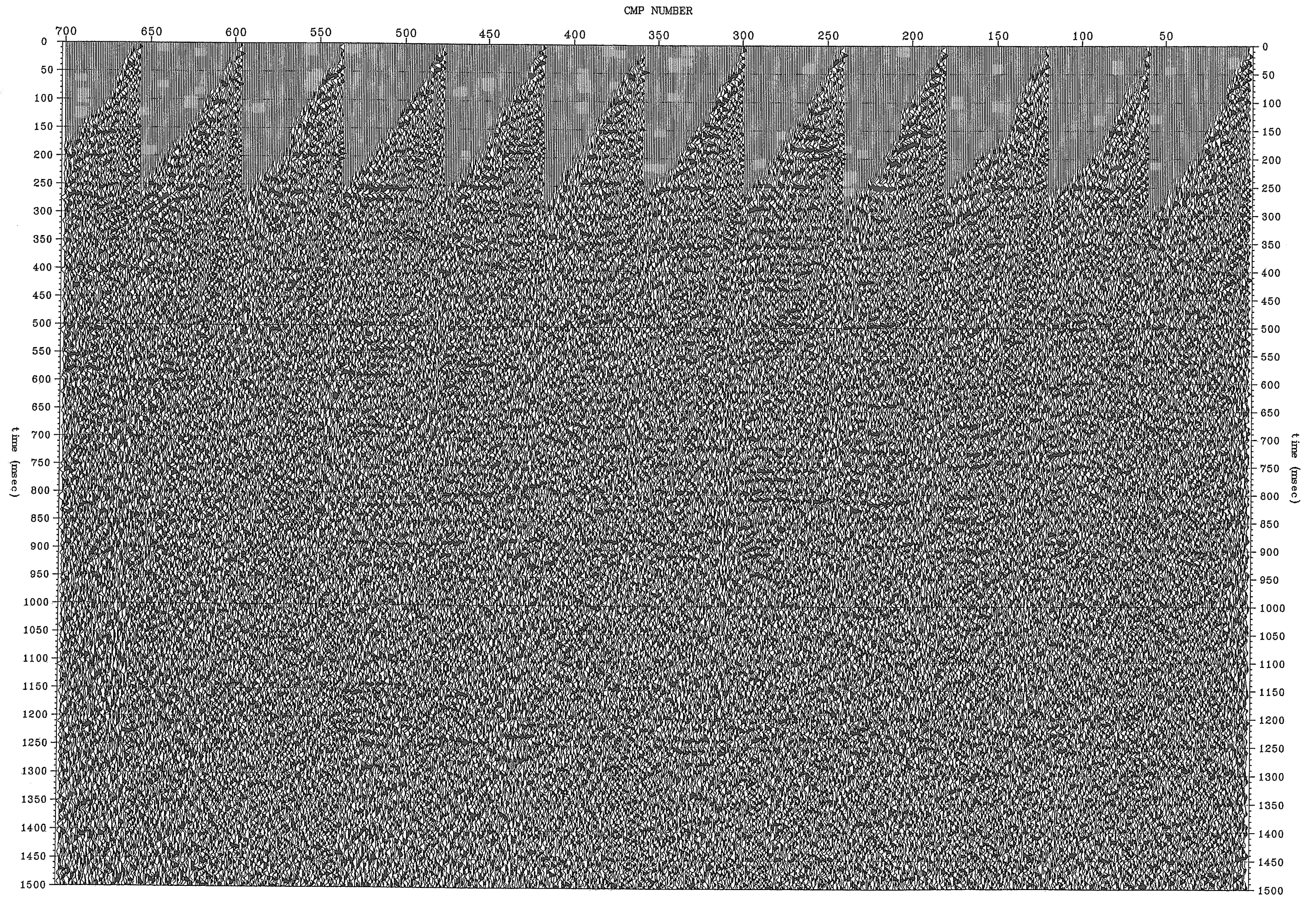
図 3. 1. 10 (5) -1 NMO補正後の 100%断面 (Line1 測線, CMP1~700)
