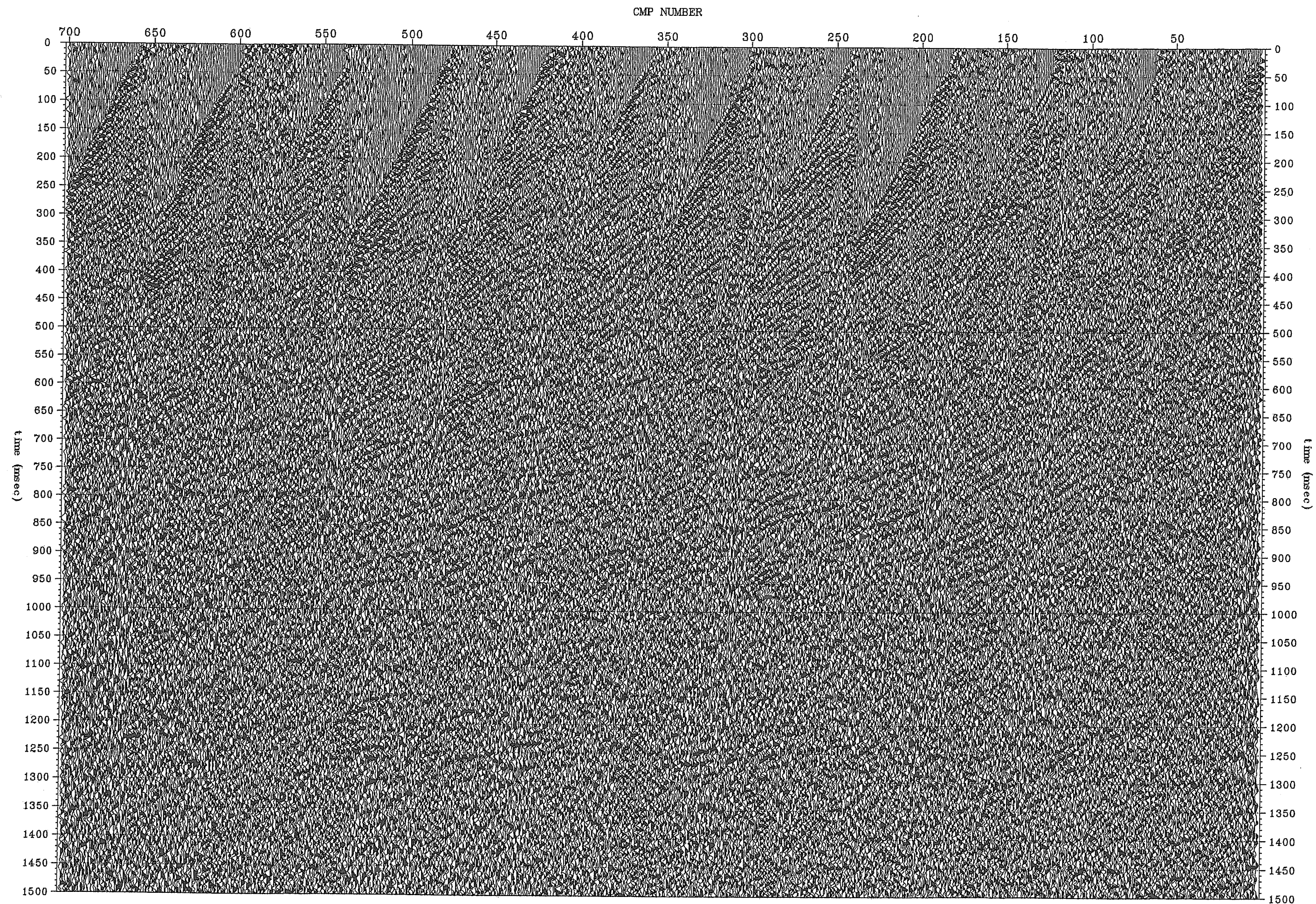
図 3. 1. 10 (3) -1 静補正後の 100%断面 (Line1 測線, CMP1~700)
