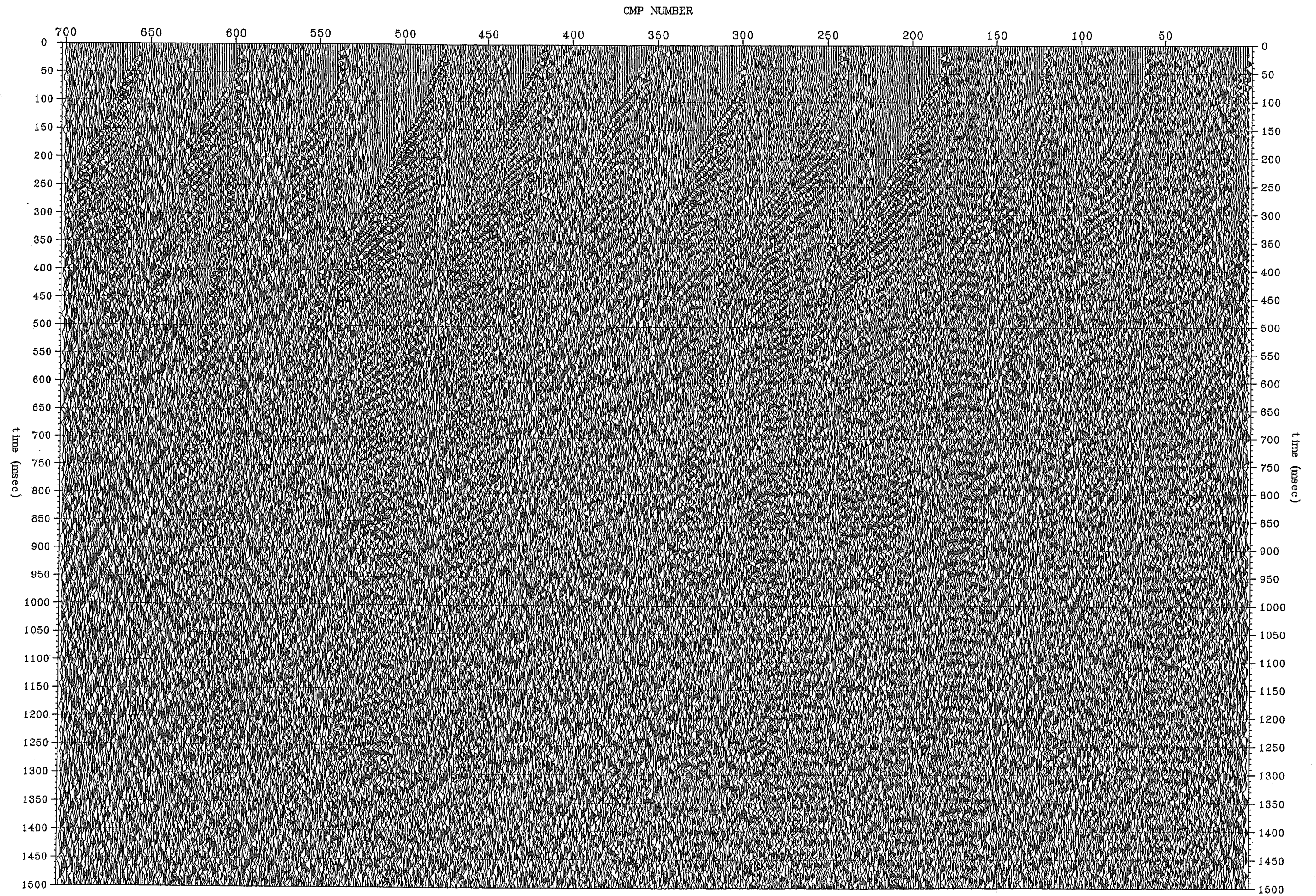
図 3. 1. 10 (2) -1 プレフィルタリング・位相補償・振幅調整後の 100%断面 (Line1 測線, CMP1~700)
