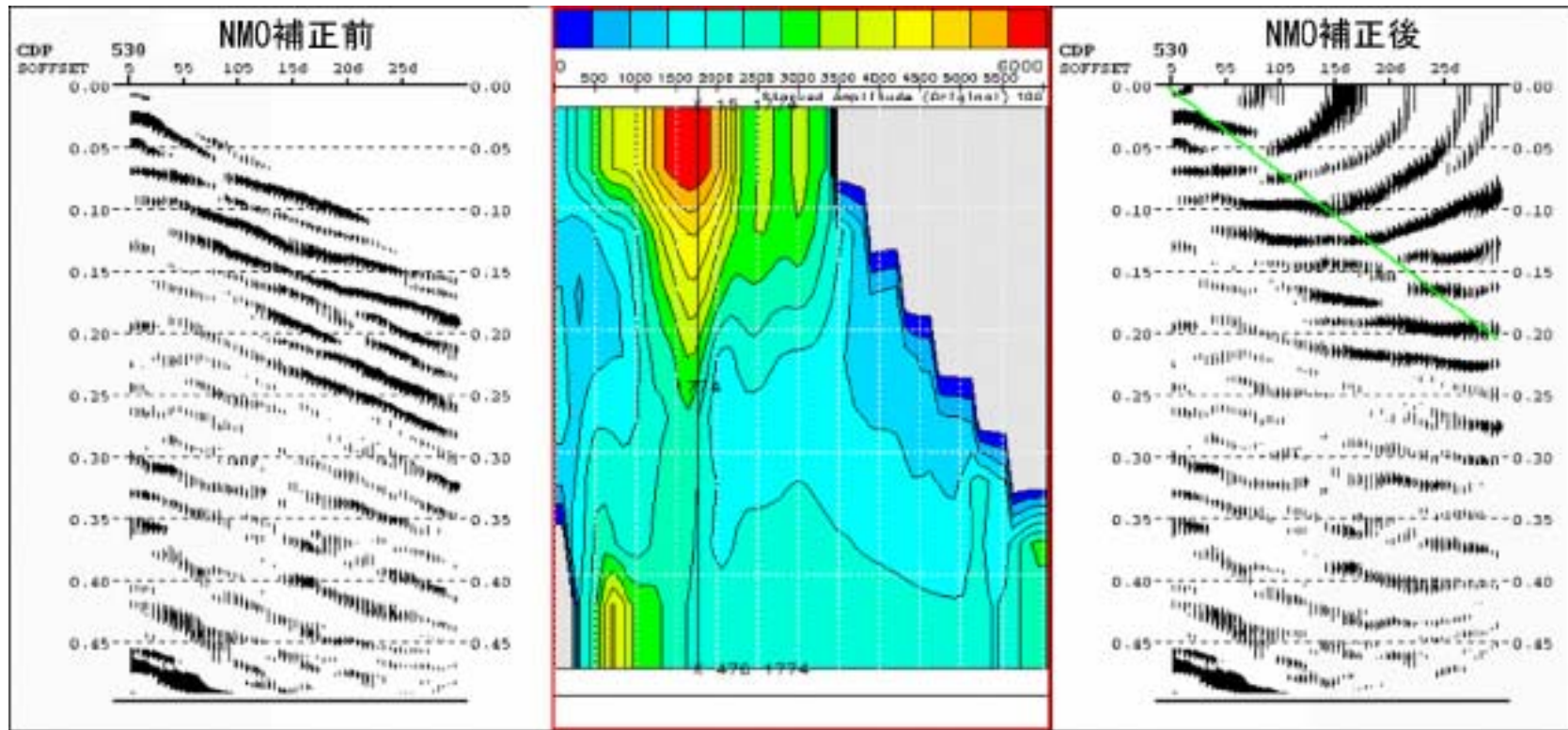
図 2-2-7 速度解析及び NMO 補正の適用 ( S 波記録 )
