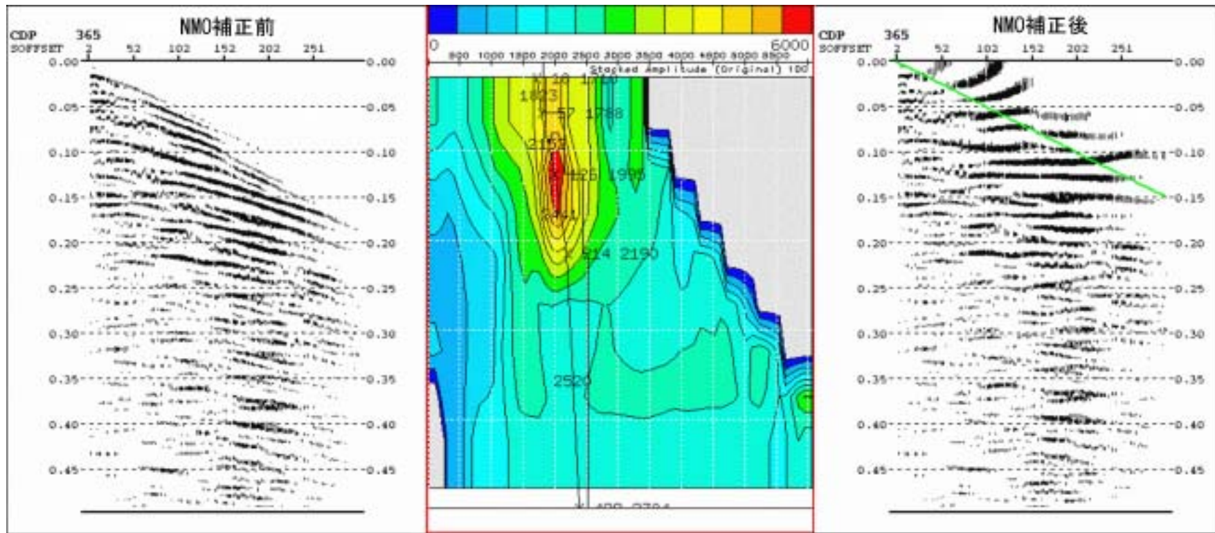
図 2-2-6 速度解析及び NMO 補正の適用 ( P 波記録 )
