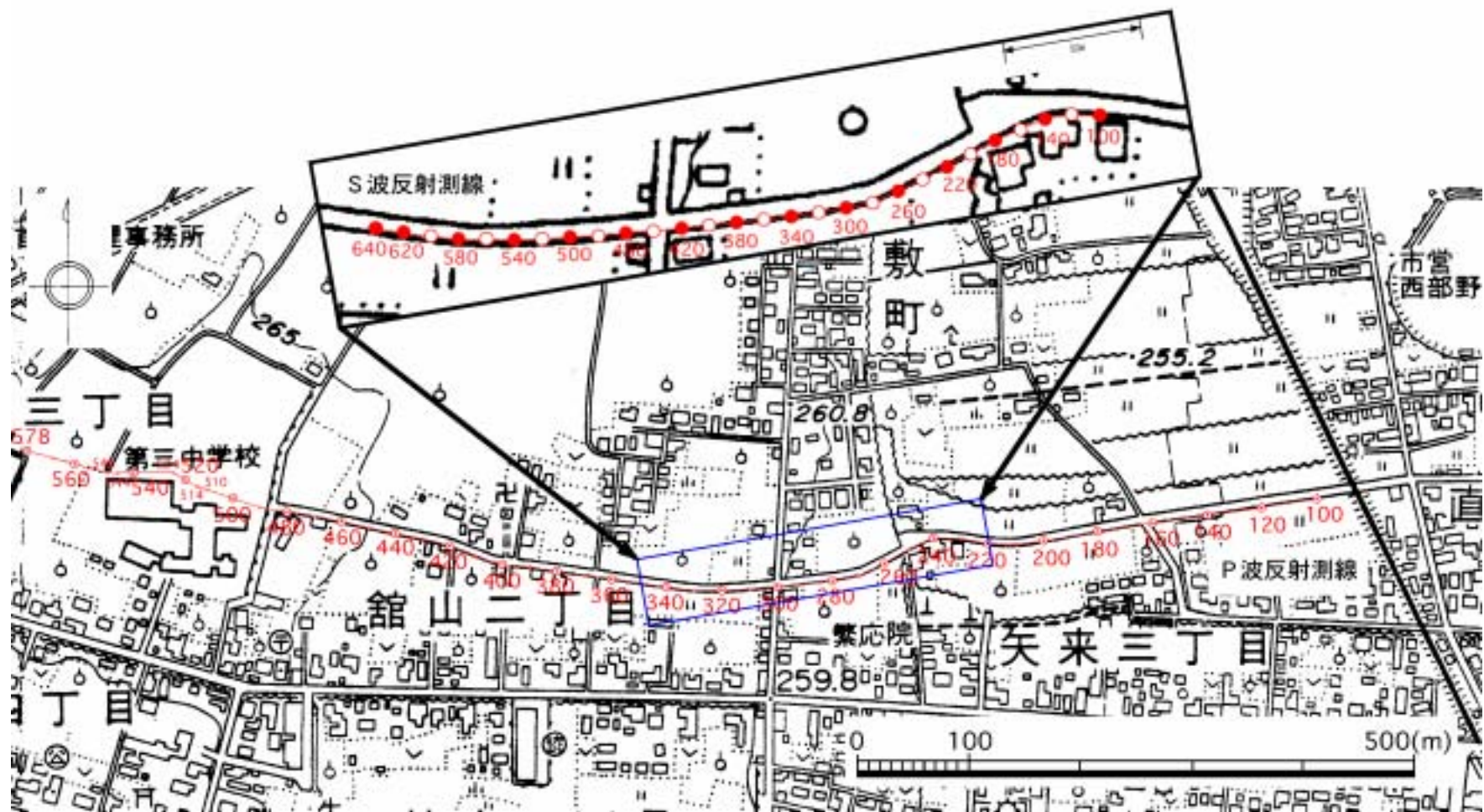
図 2-2-2 反射法探査測線図（米沢市館山地区 P 波探査測線及び S 波探査測線）
