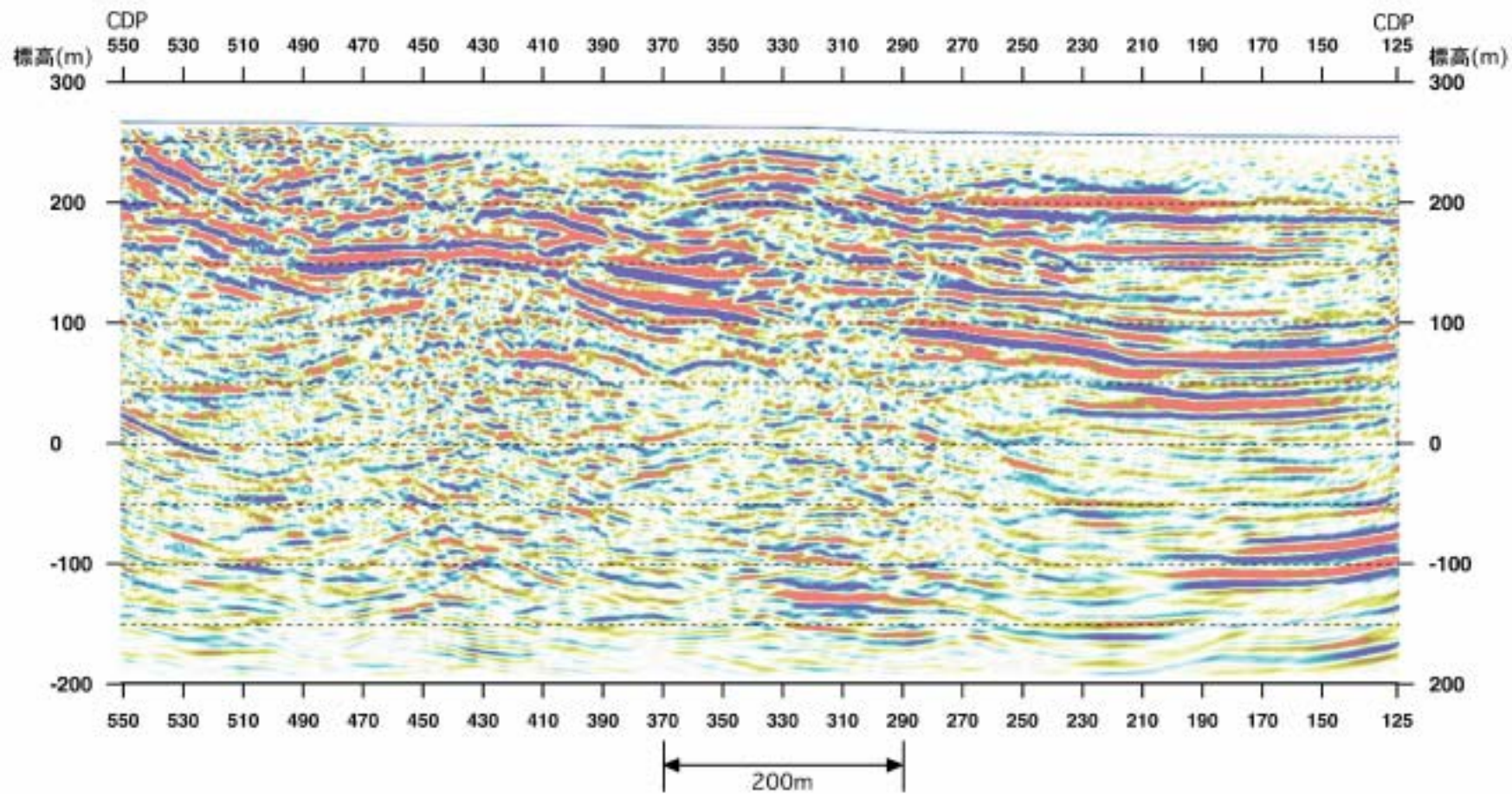
図 2-2-15 深度断面図（米沢市館山地区：P 波） （振幅値によるカラー表示）
