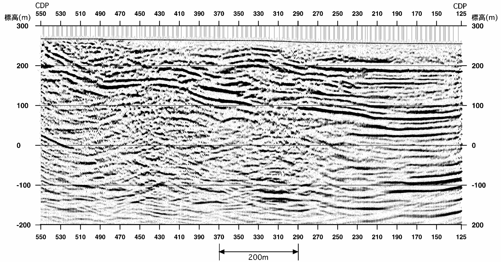
图 2-2-14 深度断面图 (米沢市館山地区:P波)
