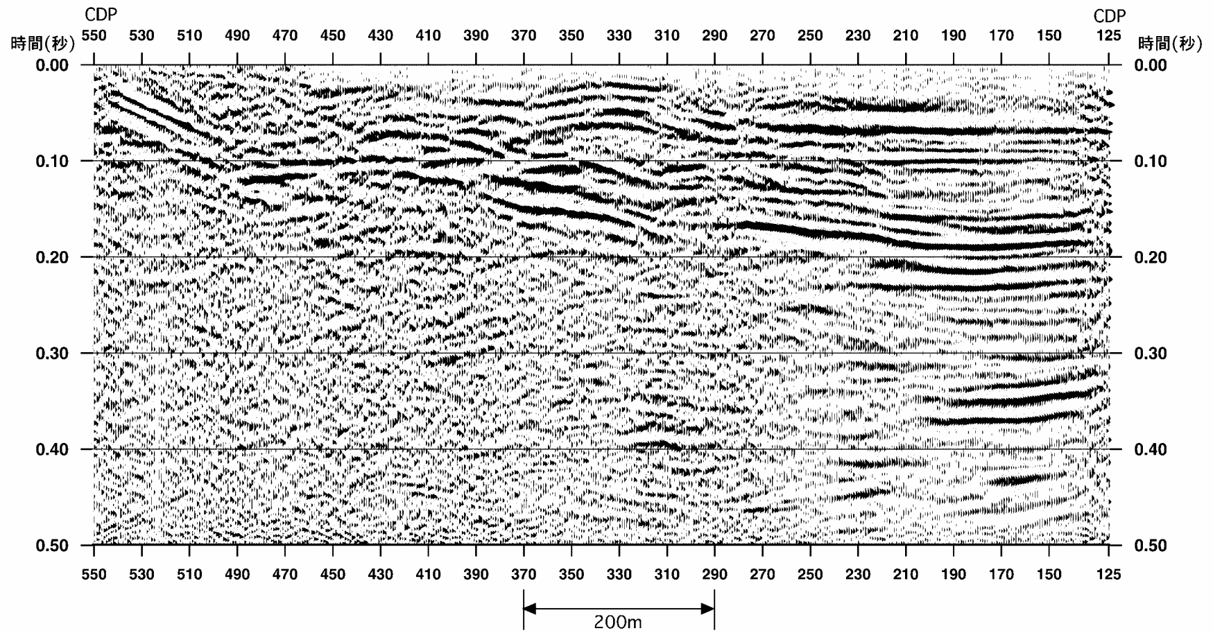
图 2-2-12 重合断面图 (米沢市館山地区:P波)
