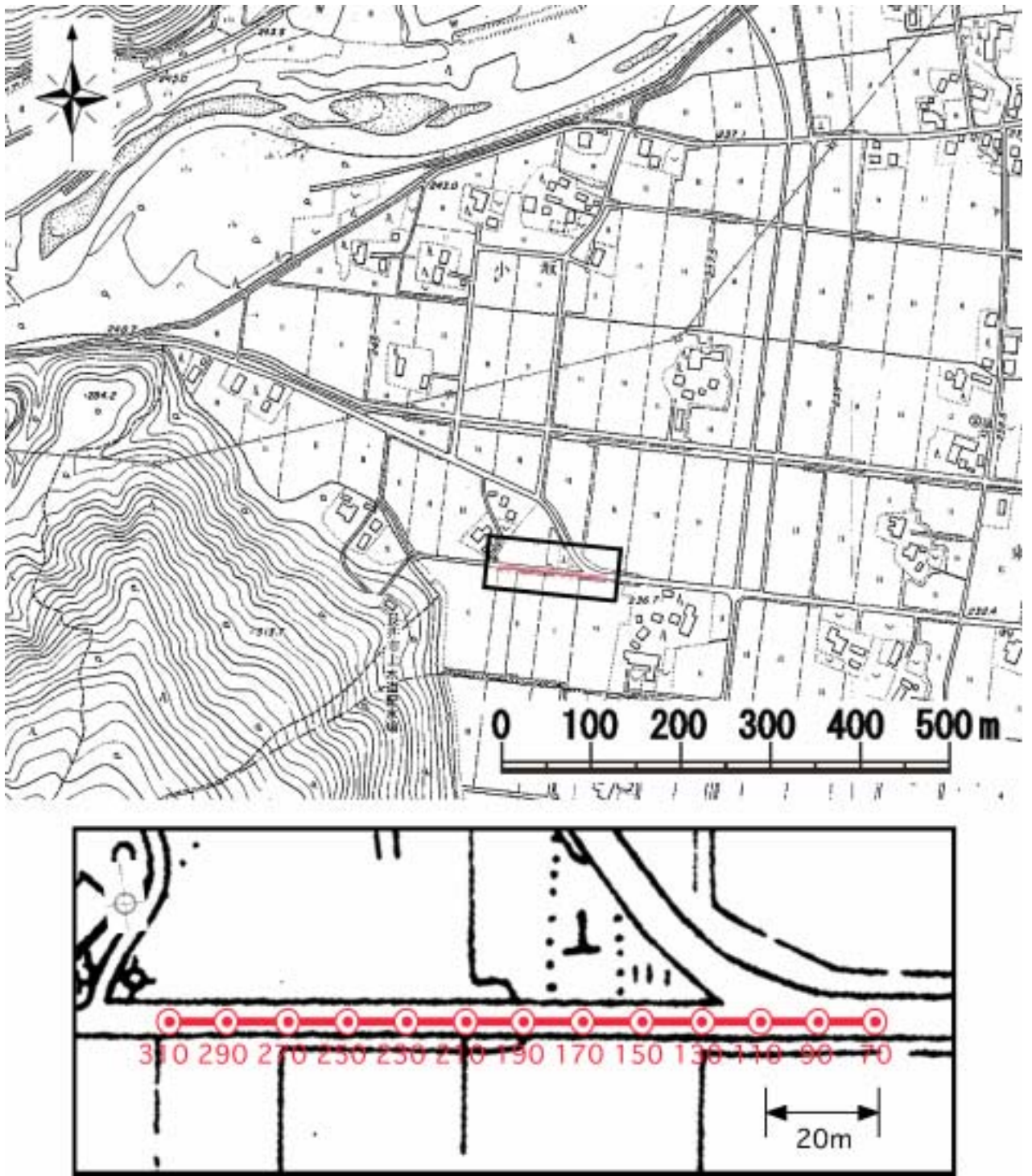
图 2-2-1 反射法探查測線図（長井市平山地区:S波）
