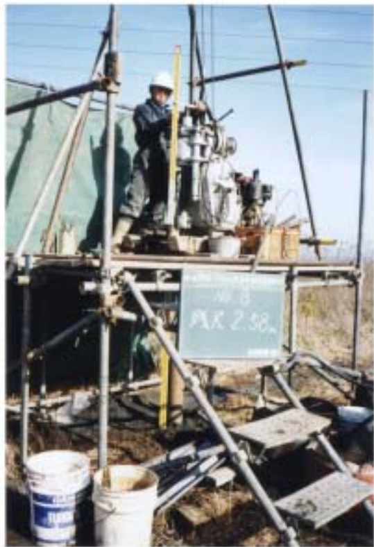
ボーリング 大野川No. 8孔
