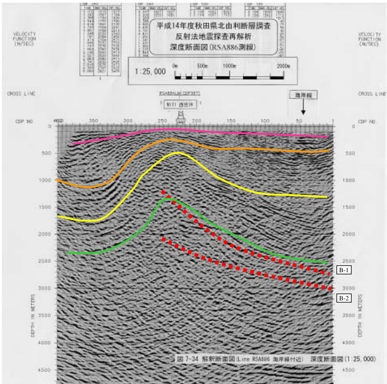
図7-34 解釈断面図(RSA886海岸線付近)
