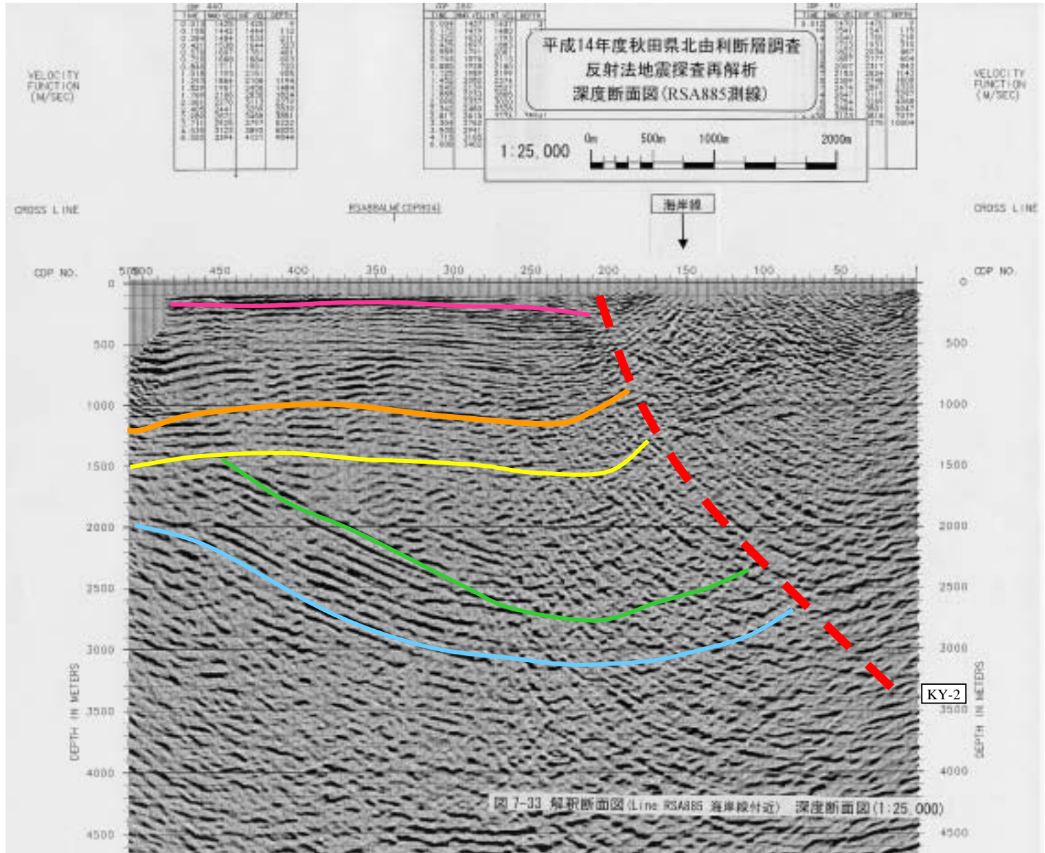
図7-33 解釈断面図(RSA885海岸線付近)
