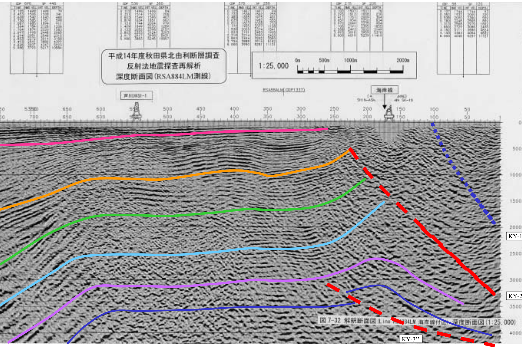
図7-32 解釈断面図(RSA884LM海岸線付近)
