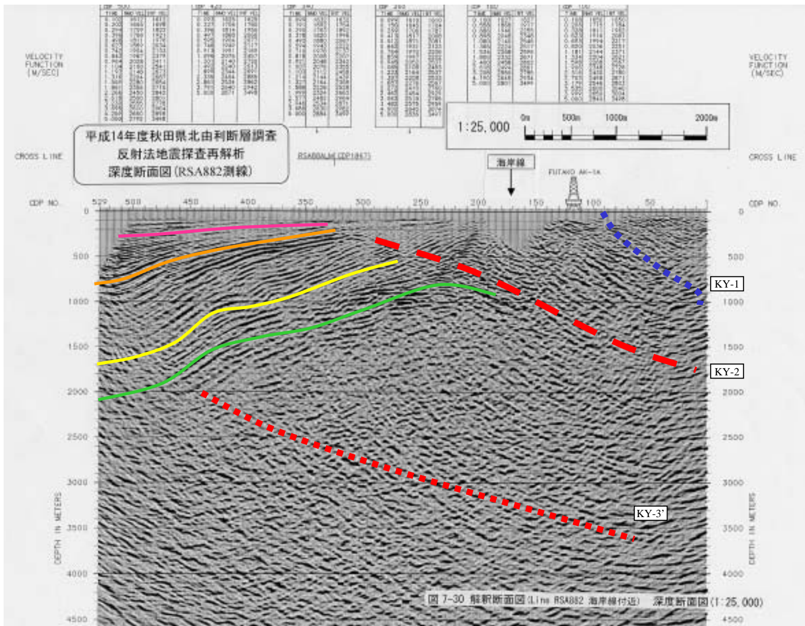
図7-30 解釈断面図(RSA882海岸線付近)
