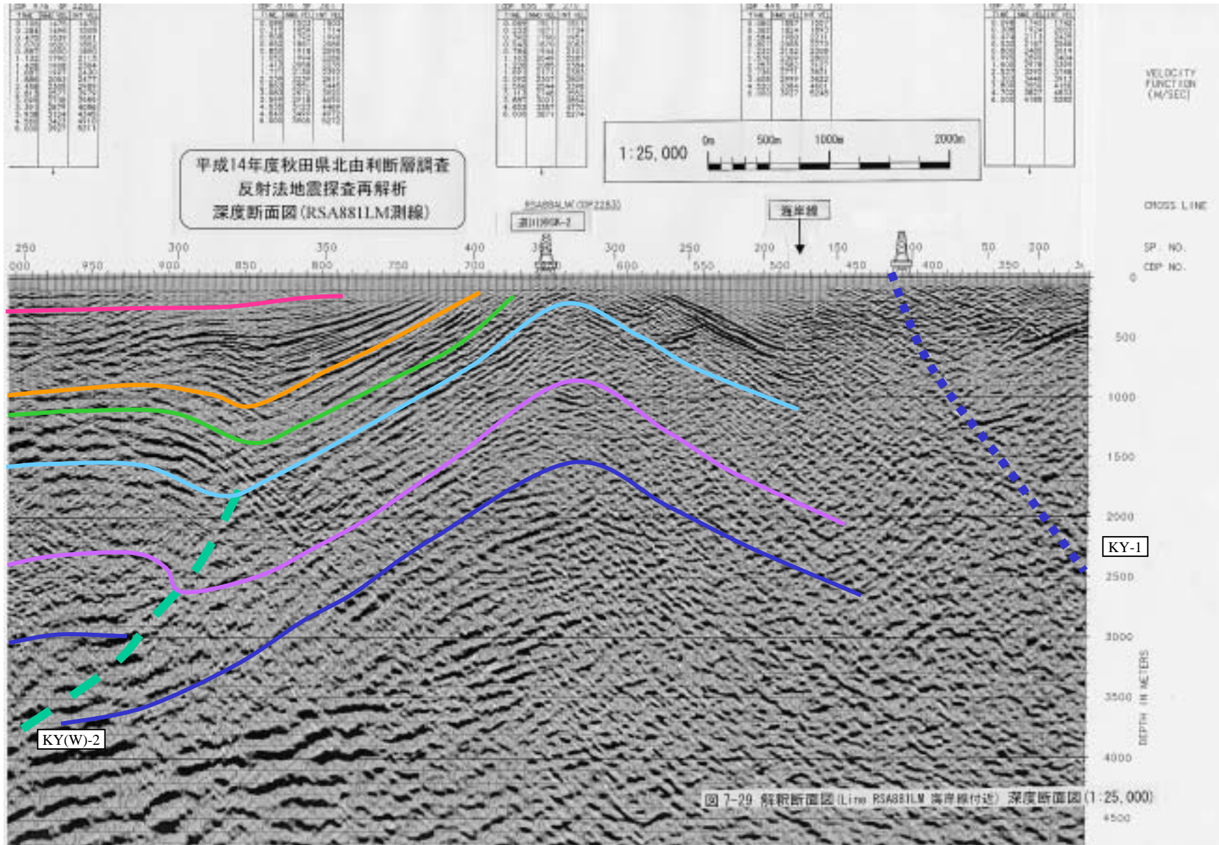
図7-29 解釈断面図(RSA881LM海岸線付近)
