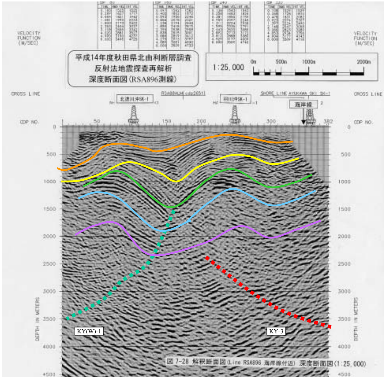
図7-28 解釈断面図(RSA896海岸線付近)
