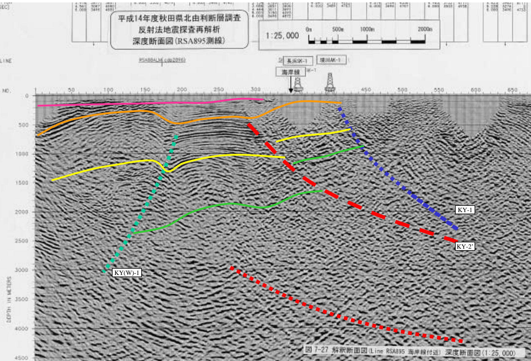
図7-27 解釈断面図(RSA895海岸線付近)
