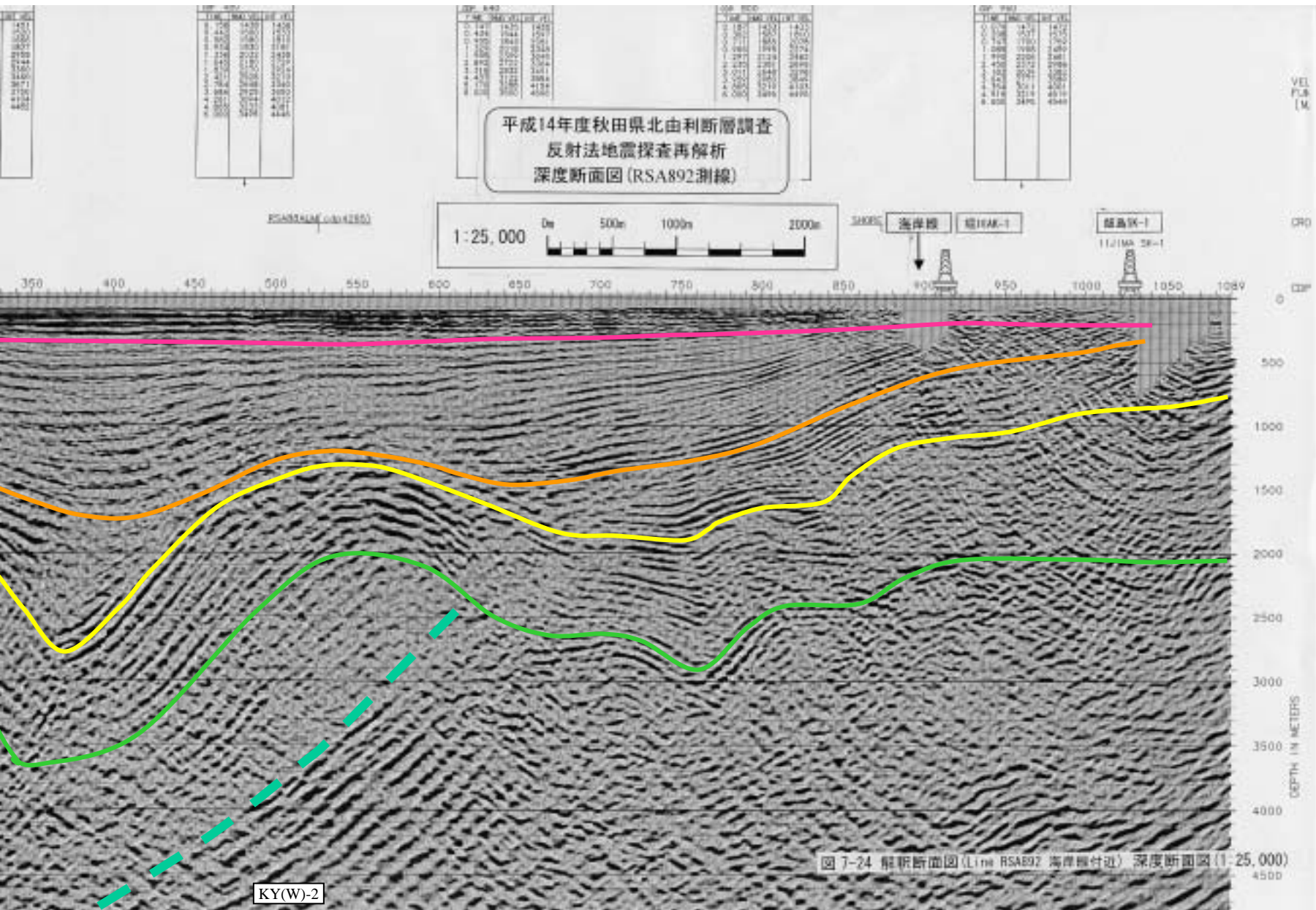
図7-24 解釈断面図(RSA892海岸線付近)
