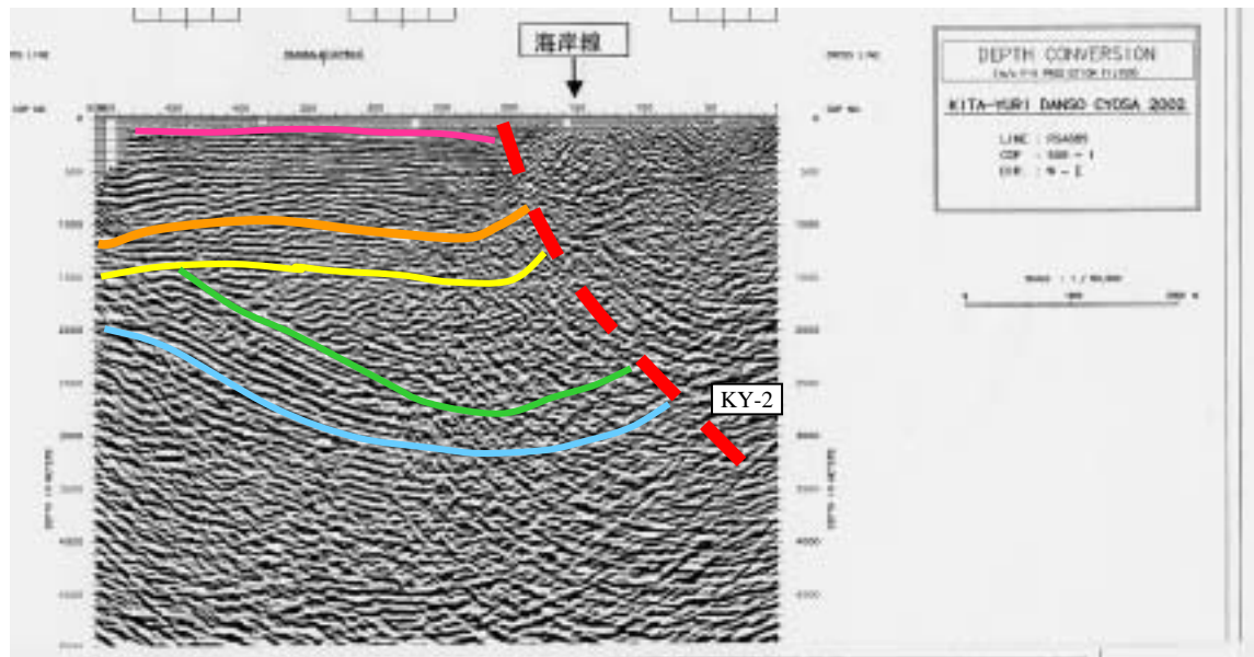
図7-23 解釈断面図(RSA885-886)
