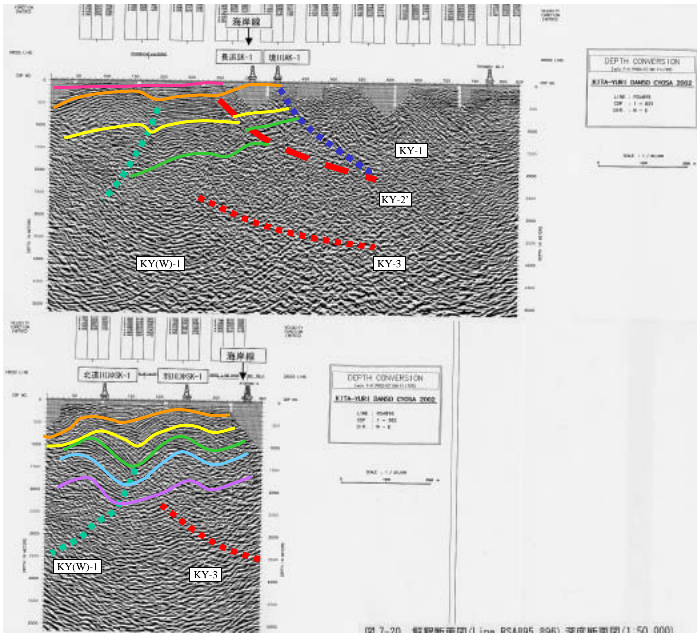
图 7-20 解释断面图(Line RSA895、896) 深度断面图(1:50,000)
