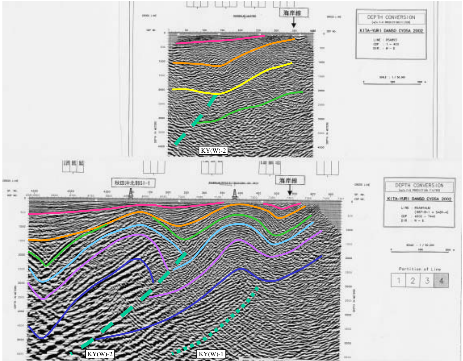
図7-19 解釈断面図(Line RSA893, 894LM) 深度断面図(1:50,000)
