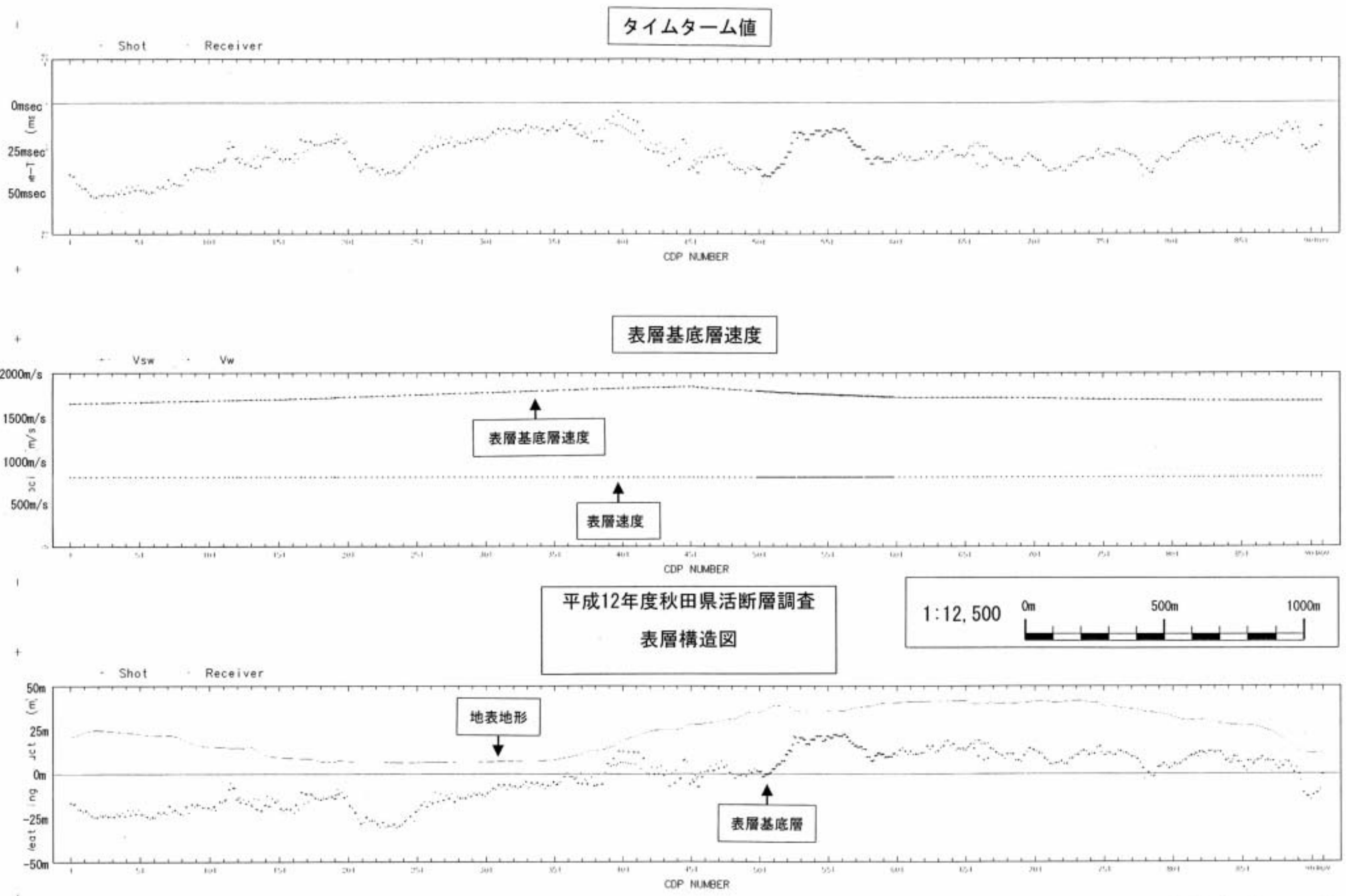
図 5-5-3 表層構造図(浅内沼測線)
